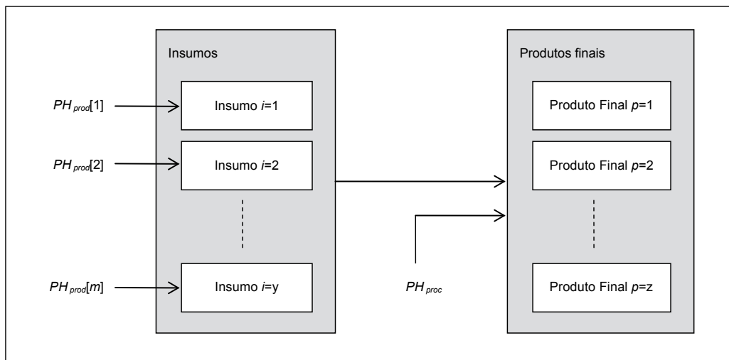
Figura 3.8 Esquematização do último passo do processo no sistema de produção do produto ‘p’. A pegada hídrica do produto final ‘p’ é calculada com base nas pegadas hídricas dos insumos e na pegada hídrica do processo quando os insumos geram os produtos finais
