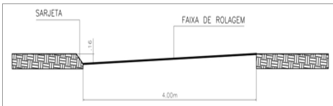
Figura 18 - Esquema da estrada considerando uma largura média de 4 metros de largura, 4% de declividade e sarjeta com 16 cm de profundidade.
