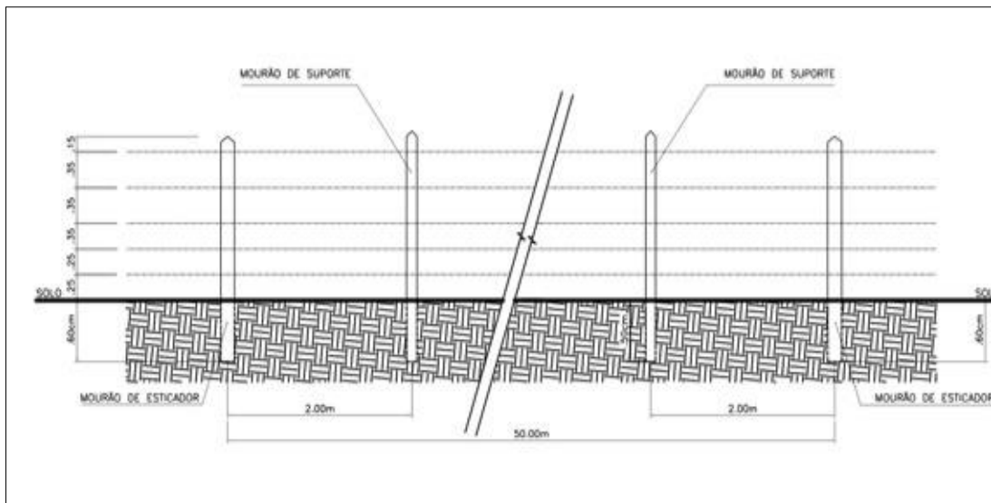
Figura 17 - Cerca mourão de eucalipto com espaçamento de 2 m e cinco fios de arame farpado.
