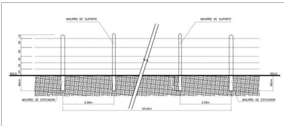
Figura 23: Cerca de mourão de eucalipto com espaçamento de 2m e cinco fios de arame farpado - ALTRAN TCBR - 2012
