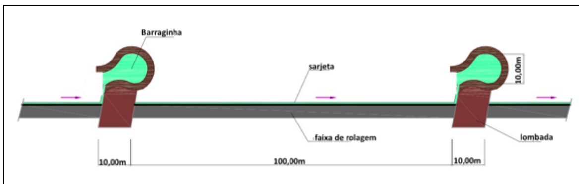
Figura 27. Situação das barragens e sarjetas e, dimensões (Altran Tcbr - 2012)
