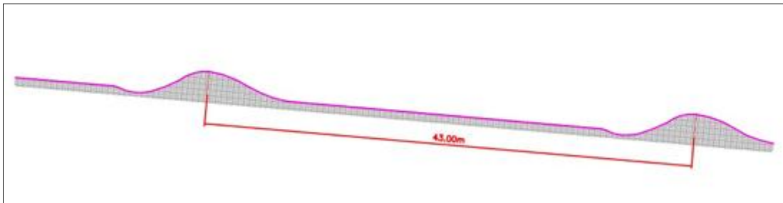
Figura 22: Distância dos terraços – Altran Tcbr - 2012
