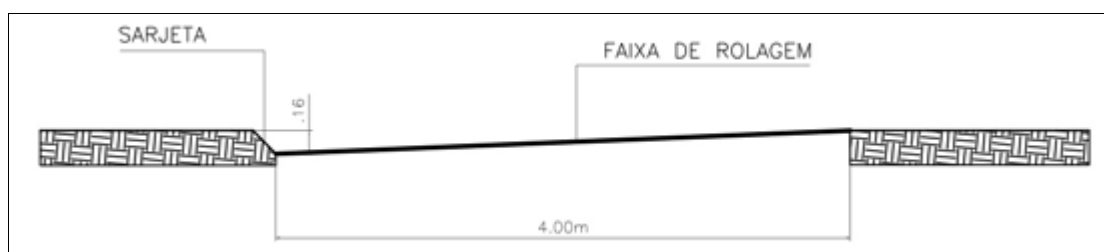
Figura 24 - Esquema da estrada considerando uma largura média de 4 m de largura, 4% de declividade e sarjeta com 16 cm de profundidade.
