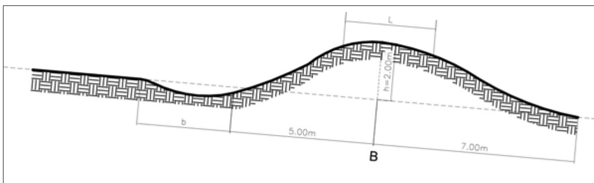
Figura 21: Corte transversal de um terraço com seção trapezoidal: B= base maior do trapézio; b= base do canal do terraço ou base menor do trapézio; h= altura do camalhão; l= largura da crista. (1985) – Altran/TCBR - 2012
