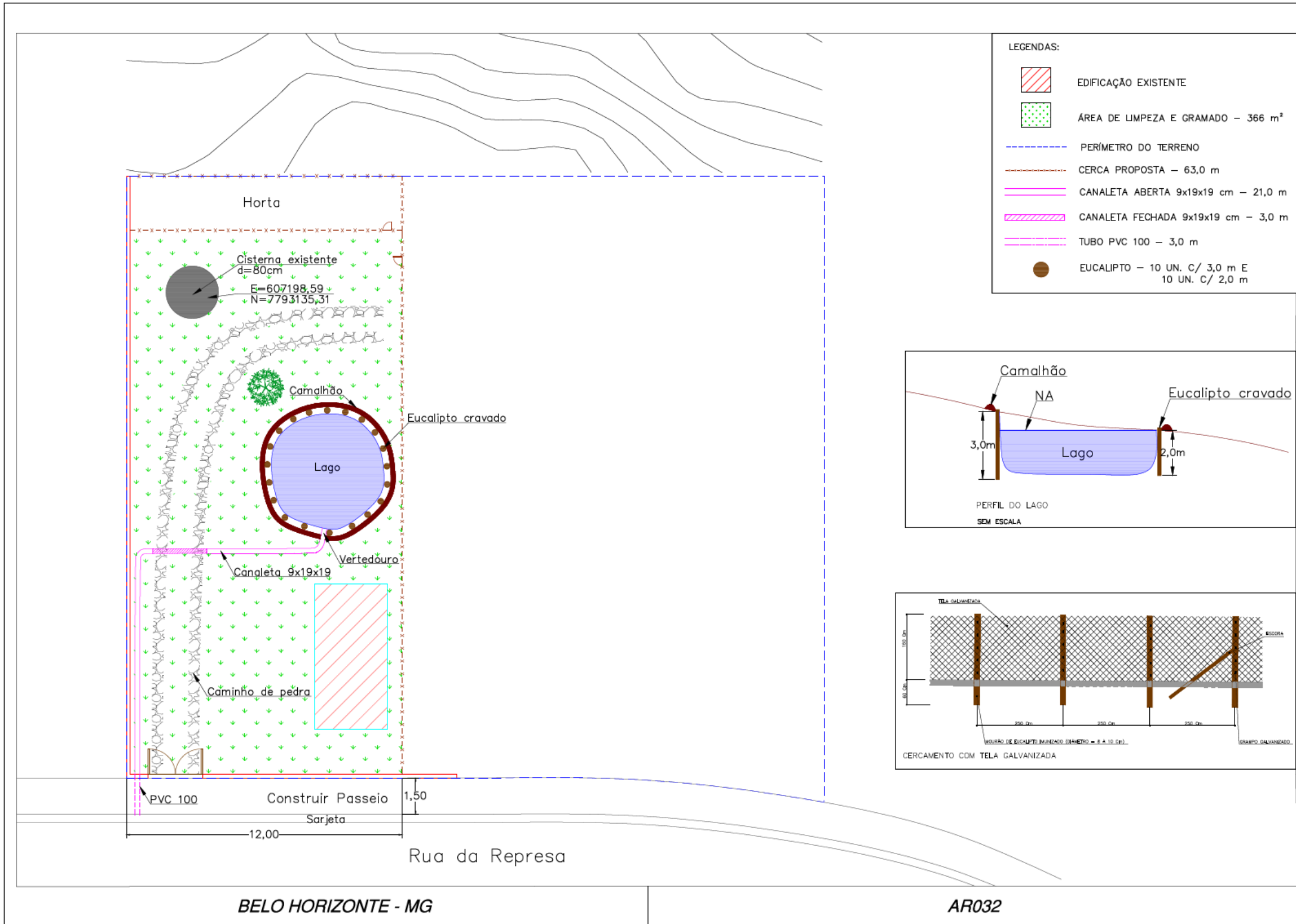
Figura 6.5 – Projeto de valorização da nascente AR-032
