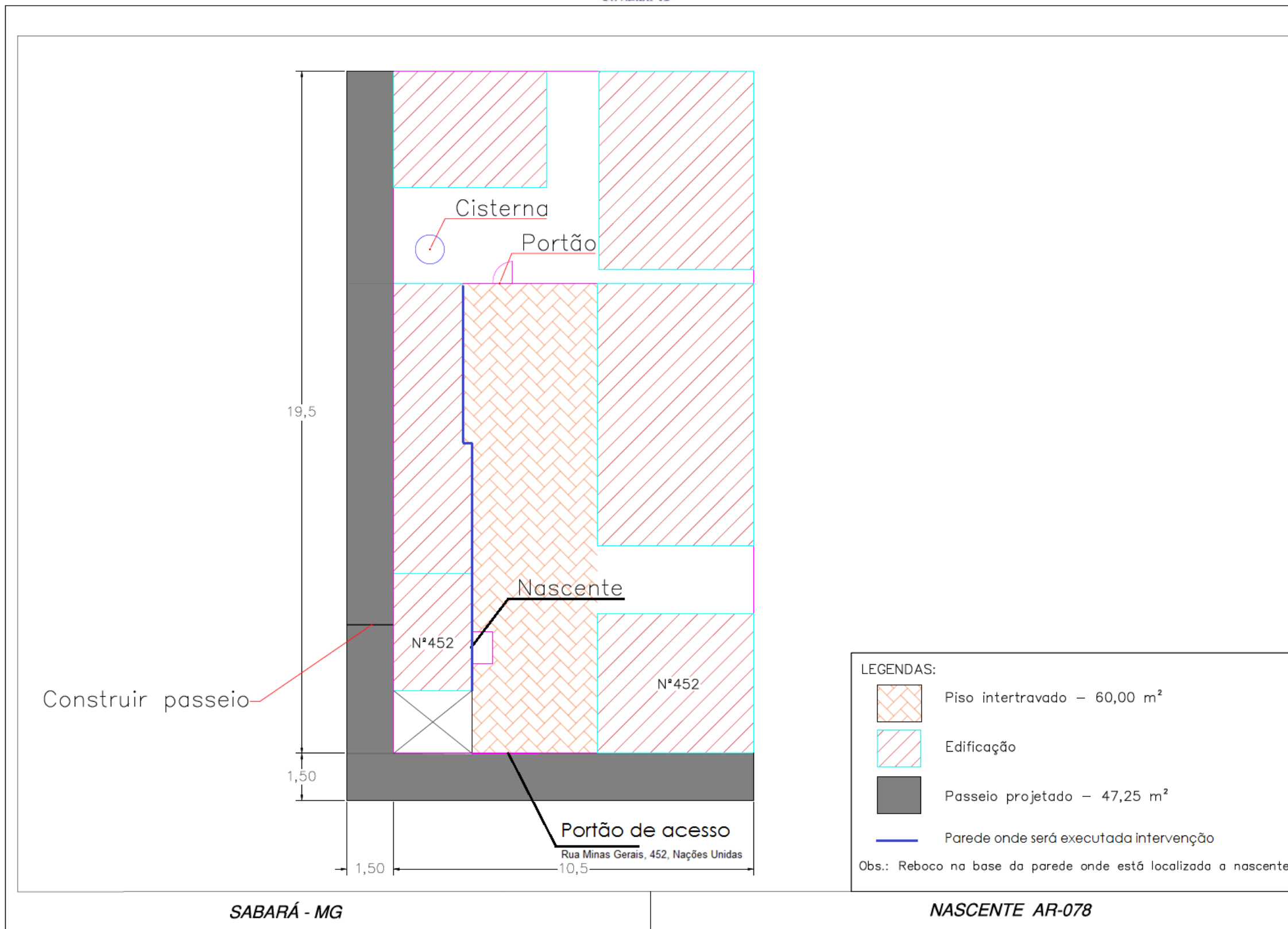
Figura 6.8 – Projeto de valorização da nascente AR-078
