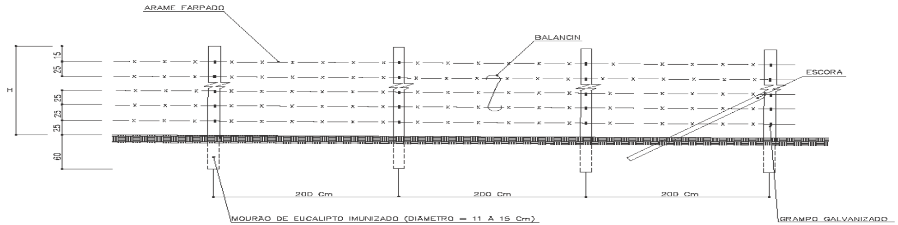
CERCAMENTO COM ARAME FARPADO
