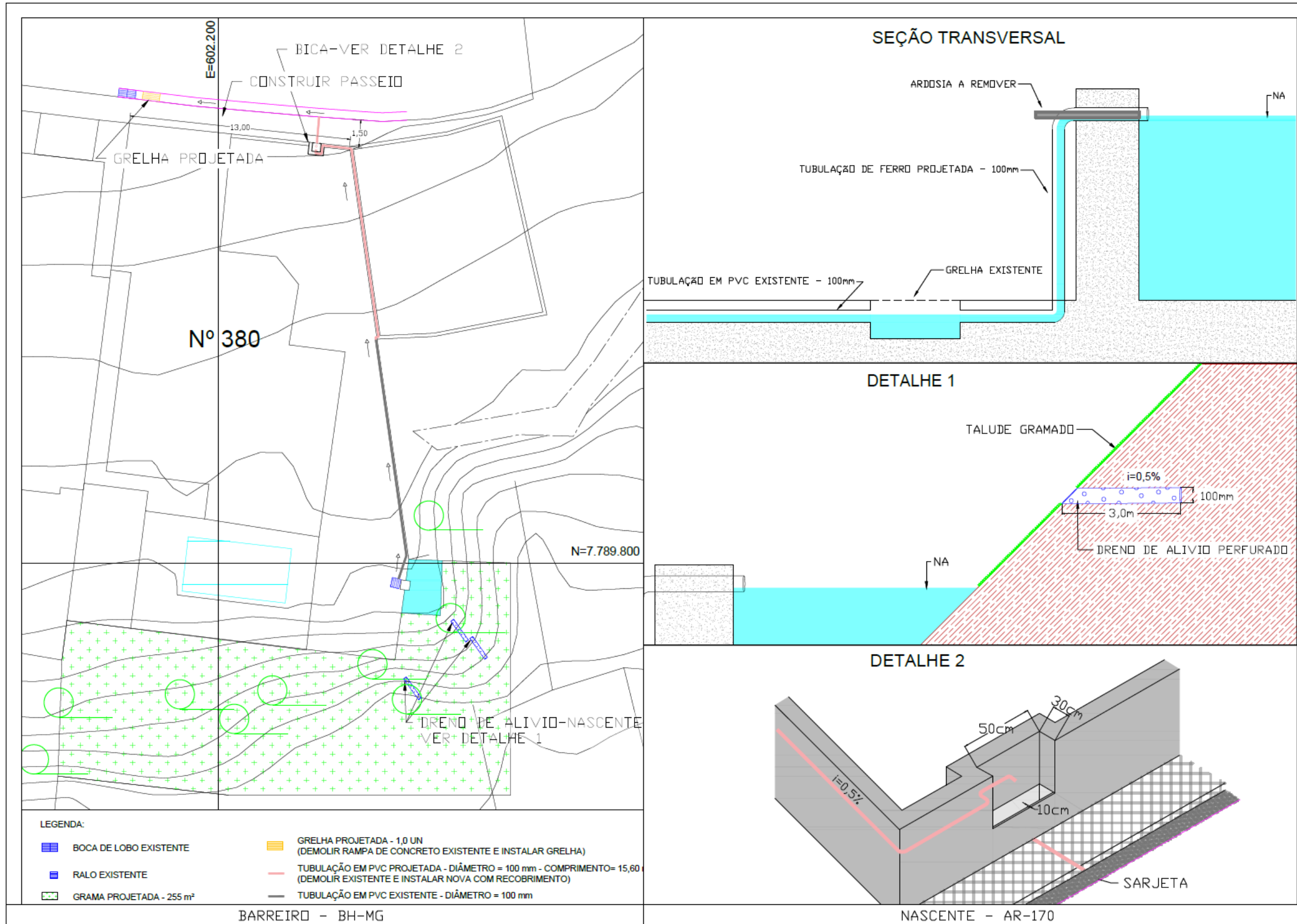
Figura 6.23 – Projeto de valorização da nascente AR-170
