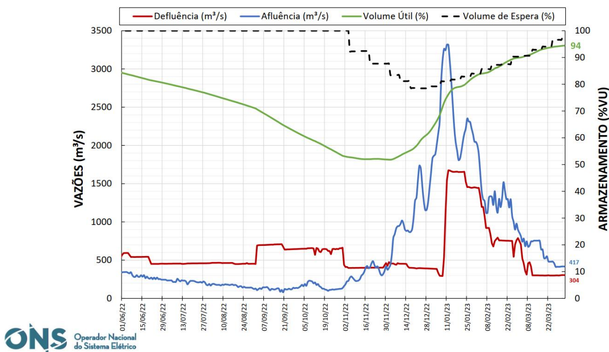
Figura 10. Regras de operação no reservatório de Três Marias até o início de abril.
