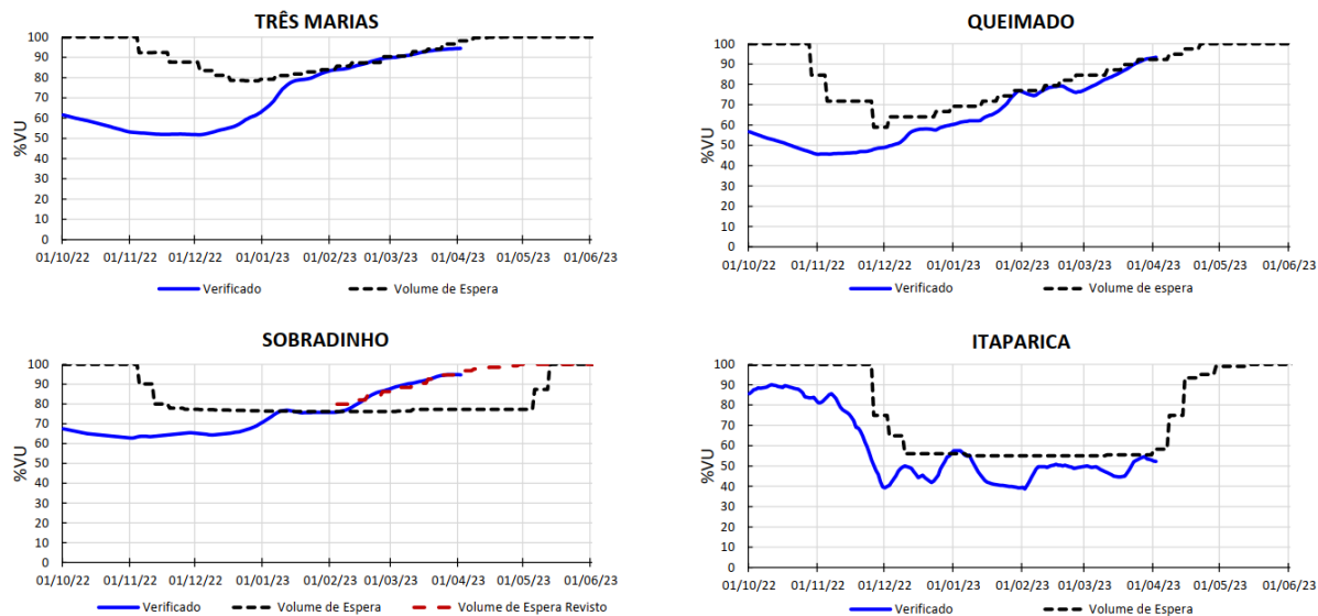
Figura 12. Volumes de espera em operação nos quatro reservatório para controle de cheias na bacia do rio São Francisco. Fonte: Apresentação técnica realizada na Quarta Reunião de Acompanhamento das condições de operação do Sistema Hídrico do Rio São Francisco em 2023, em 04 de abril de 2023.
