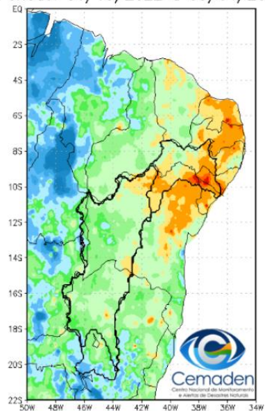
Precipitação Acumulada (mm) A.S. Período: 01/10/2022 a 03/04/2023
