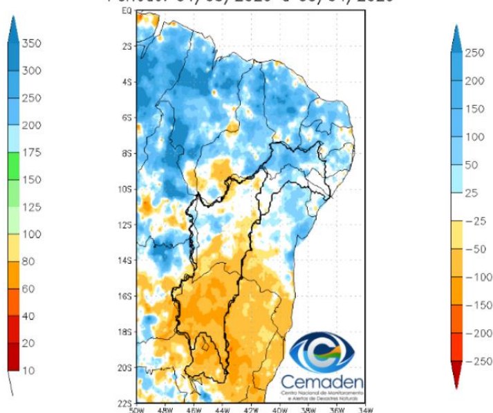
Anomalia de Precipitação (mm) A.S. Período: 04/03/2023 a 03/04/2023
