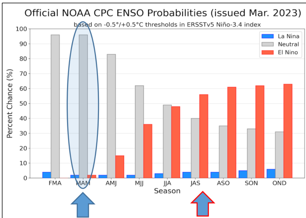
Figura 7. Caracterização de fenômeno El Nino para os próximos trimestres.
