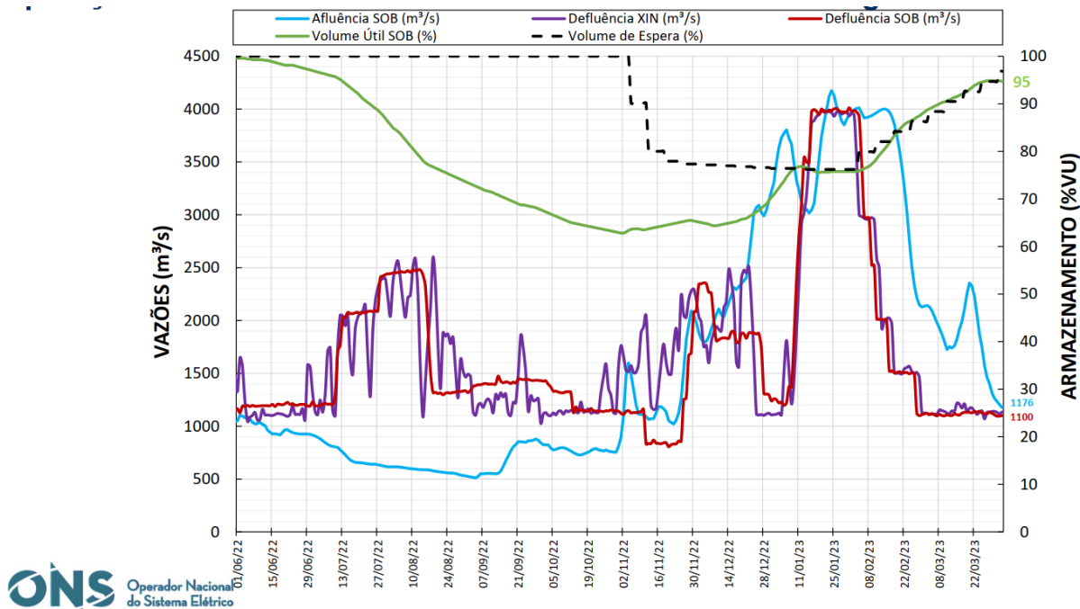
Figura 11. Regras de operação nos reservatórios de Sobradinho e Xingó até o início de abril. Fonte: Apresentação técnica realizada na Quarta Reunião de Acompanhamento das condições de operação do Sistema Hídrico do Rio São Francisco em 2023, em 04 de abril de 2023.
