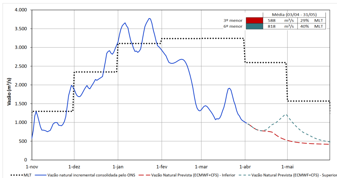
Figura 14. Vazão natural afluente no reservatório de Sobradinho para o mês de abril de 2023. Fonte: Apresentação técnica realizada na Quarta Reunião de Acompanhamento das condições de operação do Sistema Hídrico do Rio São Francisco em 2023, em 04 de abril de 2023.
