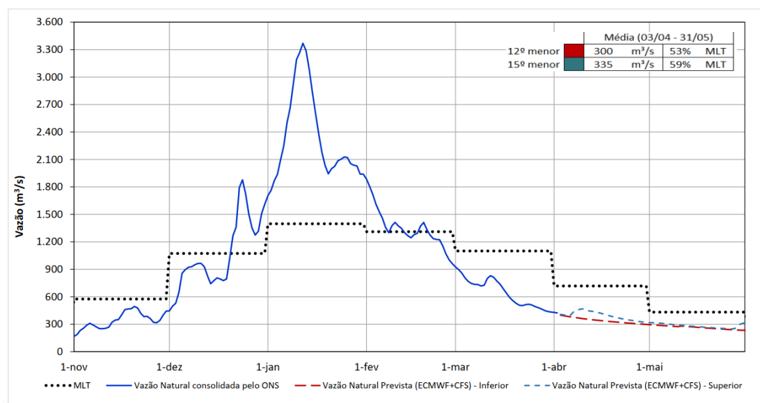
Figura 13. Vazão natural afluente no reservatório de Três Marias para o mês de abril de 2023. Fonte: Apresentação técnica realizada na Quarta Reunião de Acompanhamento das condições de operação do Sistema Hídrico do Rio São Francisco em 2023, em 04 de abril de 2023.
