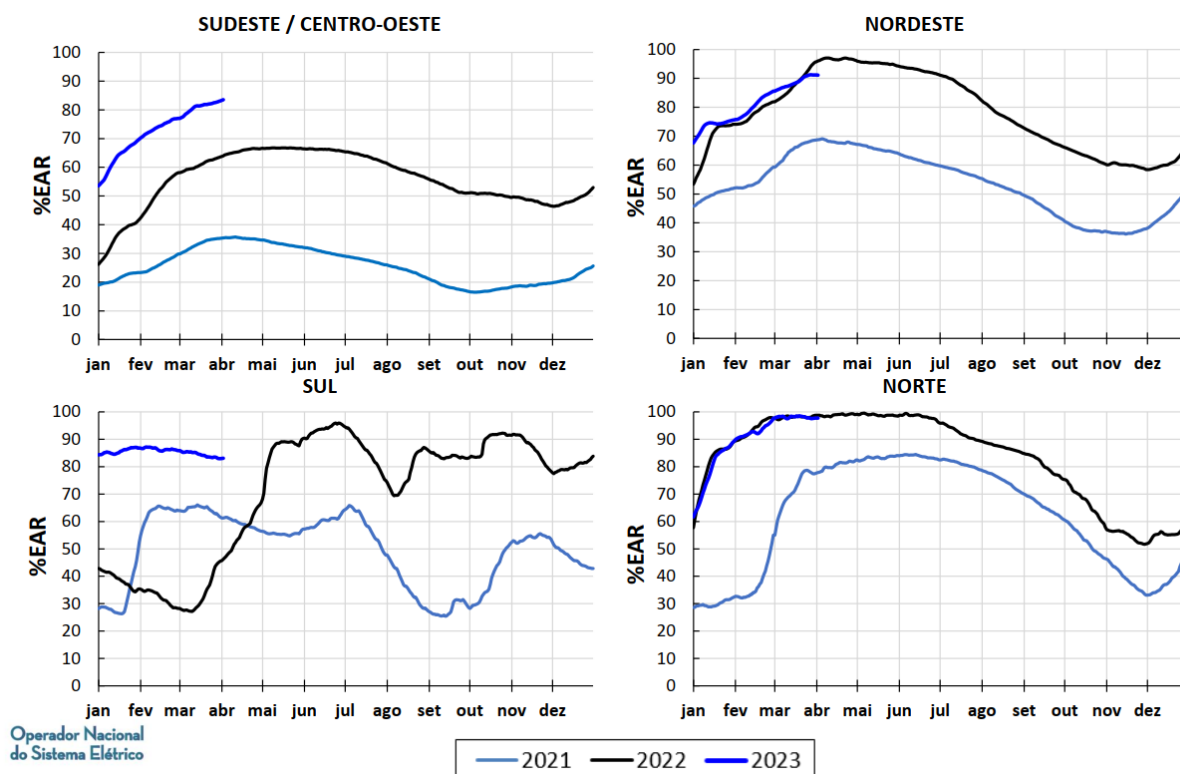
Figura 8. Volume acumulado nos reservatórios do SIN.
