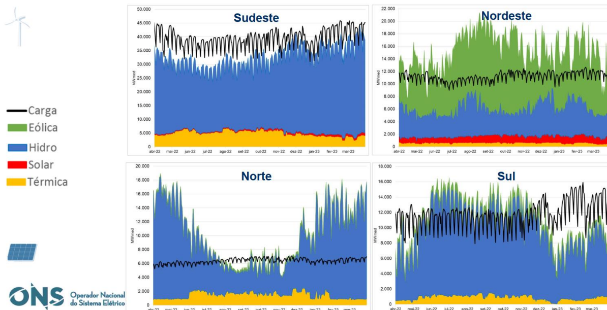
Figura 9. Necessidade de carga e geração acumulada no SIN.
