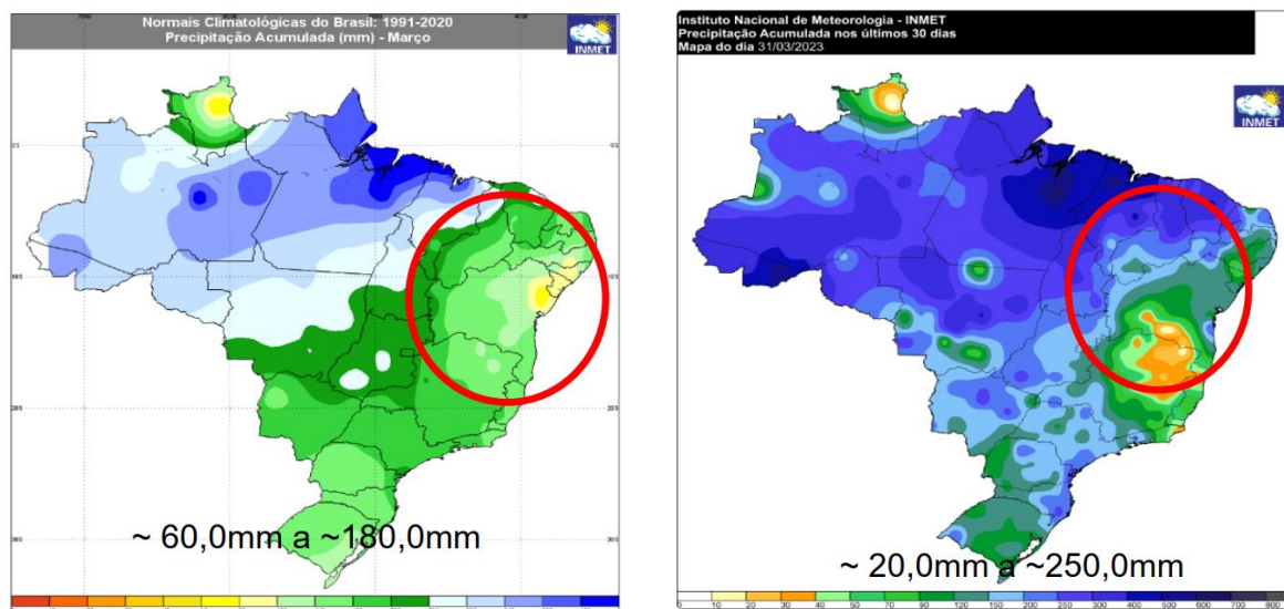
Figura 1. Normal climatológica para precipitações em março (esquerda) e volume de precipitação acumulado no mês de março de 2023 na região Nordeste do Brasil.
