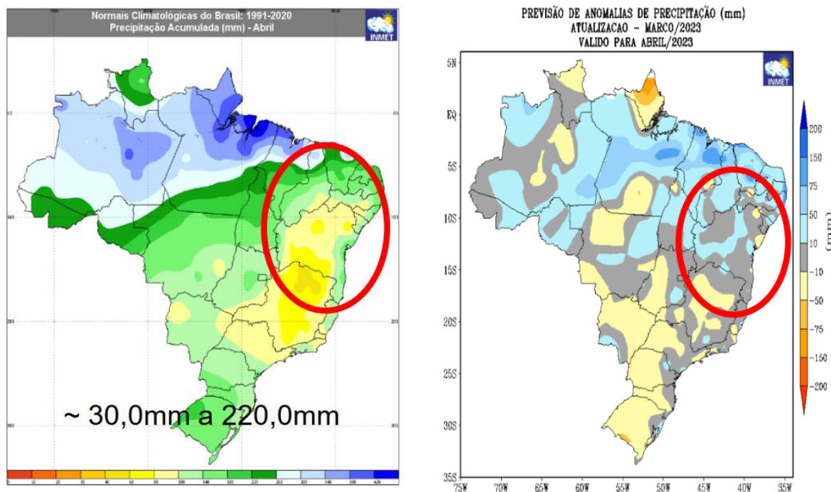
Figura 2. Normais climatológicas de precipitação em abril e previsão de anomalias de precipitação para a região Nordeste do Brasil no mês de abril de 2023.
