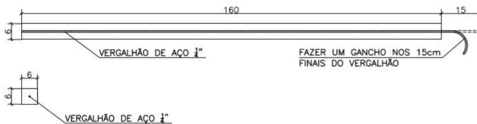
Figura 6.5 – Detalhes – Caibros da cobertura
