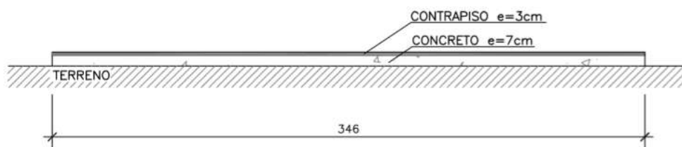
Figura 6.7 – Corte – Laje do piso Fonte: COBRAPE (2021)
