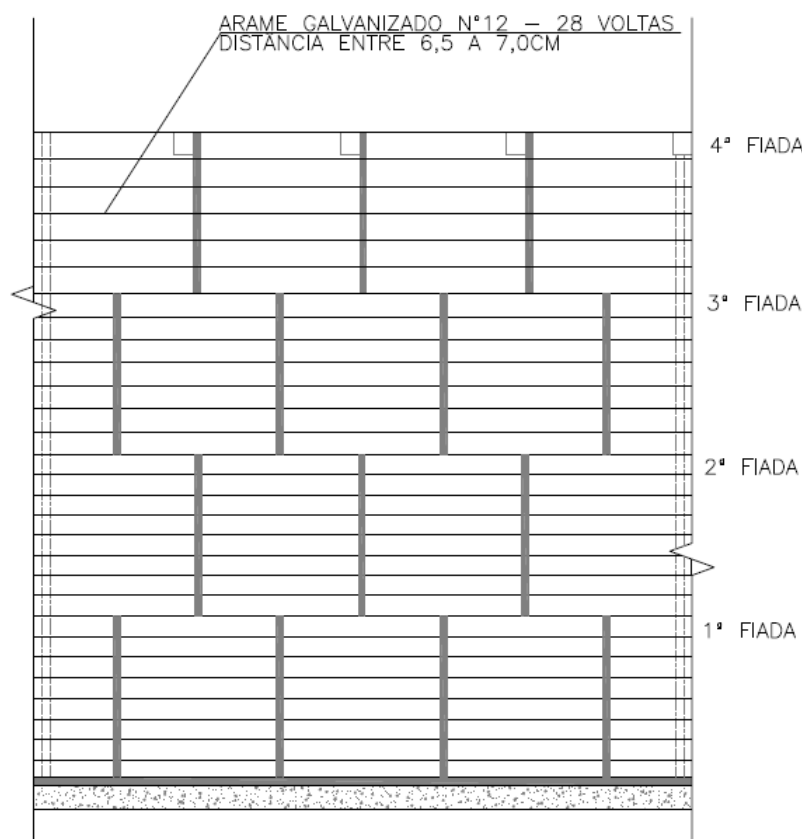
Figura 6.9 – Amarração da parede Fonte: COBRAPE (2021)
