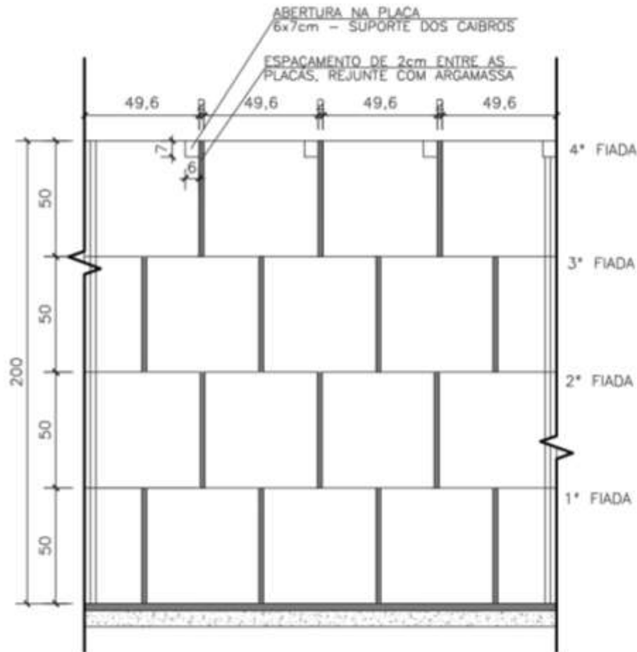
Figura 6.8 – Paginação da parede Fonte: COBRAPE (2021)
