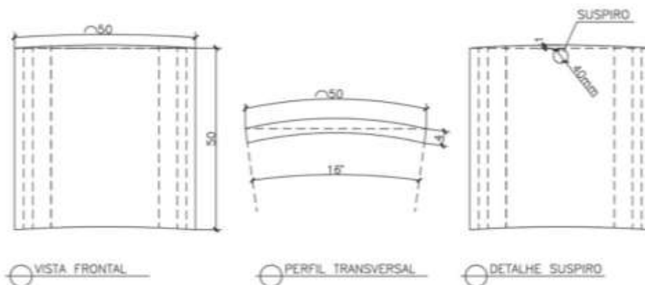
Figura 6.2 – Detalhes das Placas da parede Fonte: COBRAPE (2021)
