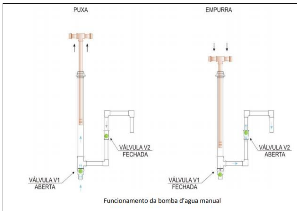
Figura 6.26 - Funcionamento da Bomba Manual
