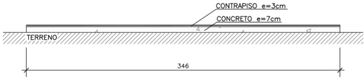
Figura 6.7 – Corte – Laje do piso
