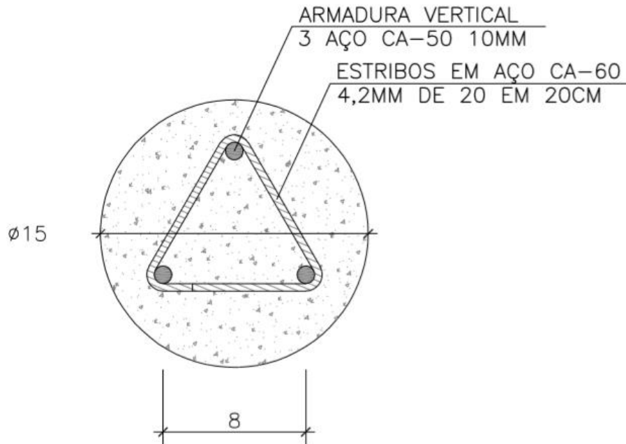
Figura 6.23 - Corte – Seção transversal do pilar central
