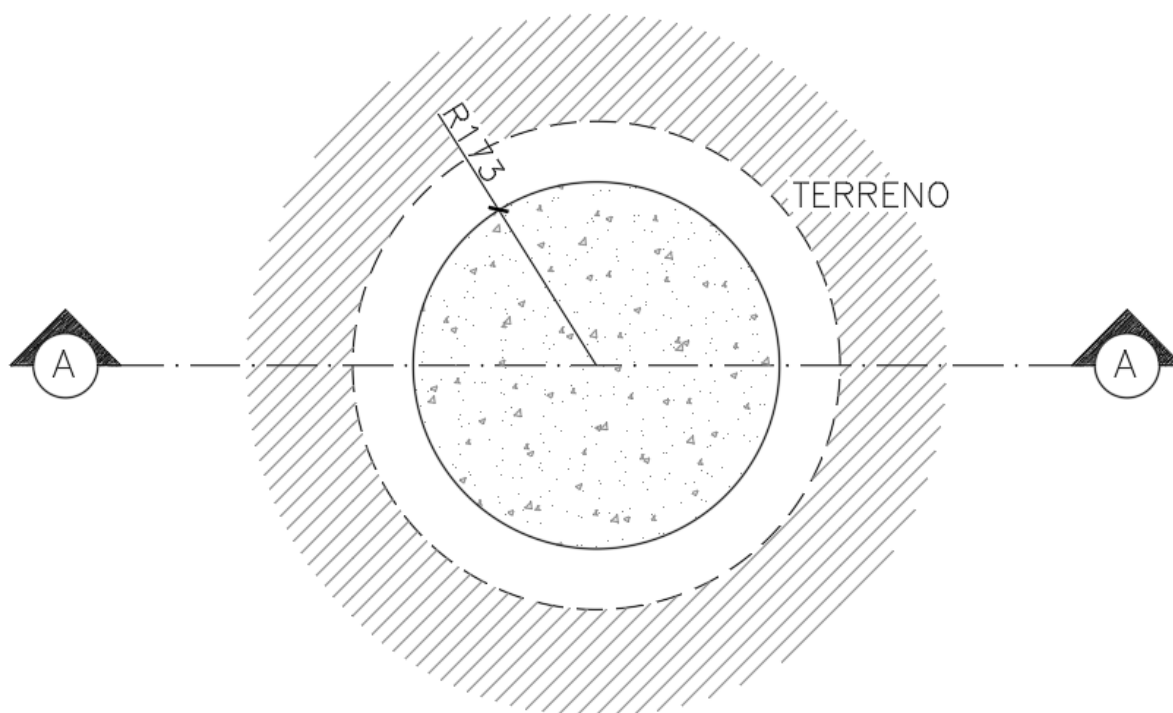
Figura 6.6 – Planta – Laje do piso
