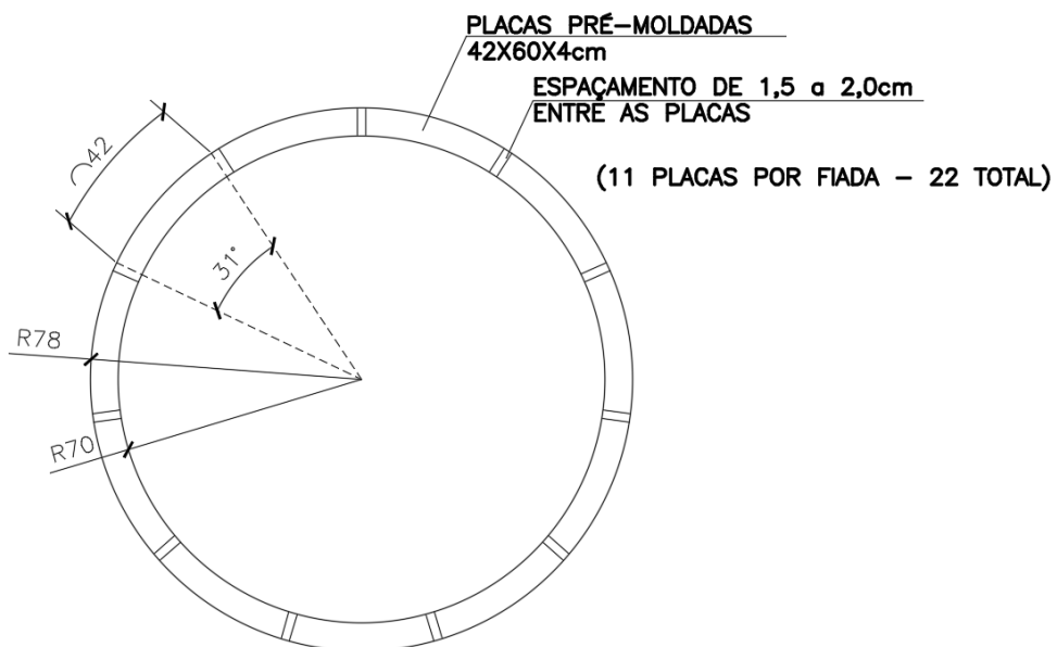
Figura 6.31 - Paredes em placas cimentícias das caixas de sedimentação Fonte: COBRAPE (2021)
