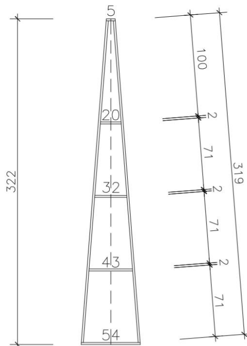
Figura 6.14 – Gabarito – Placas da cobertura
