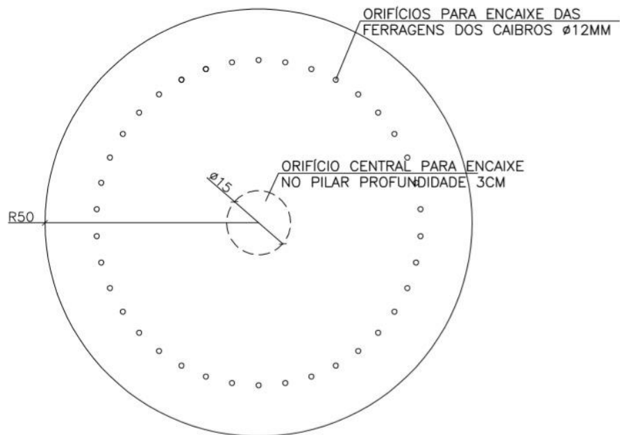
Figura 6.24 - Detalhe da coroa para suporte dos caibros
