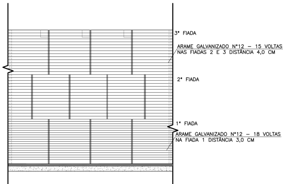
Figura 6.21 - Amarração da parede
