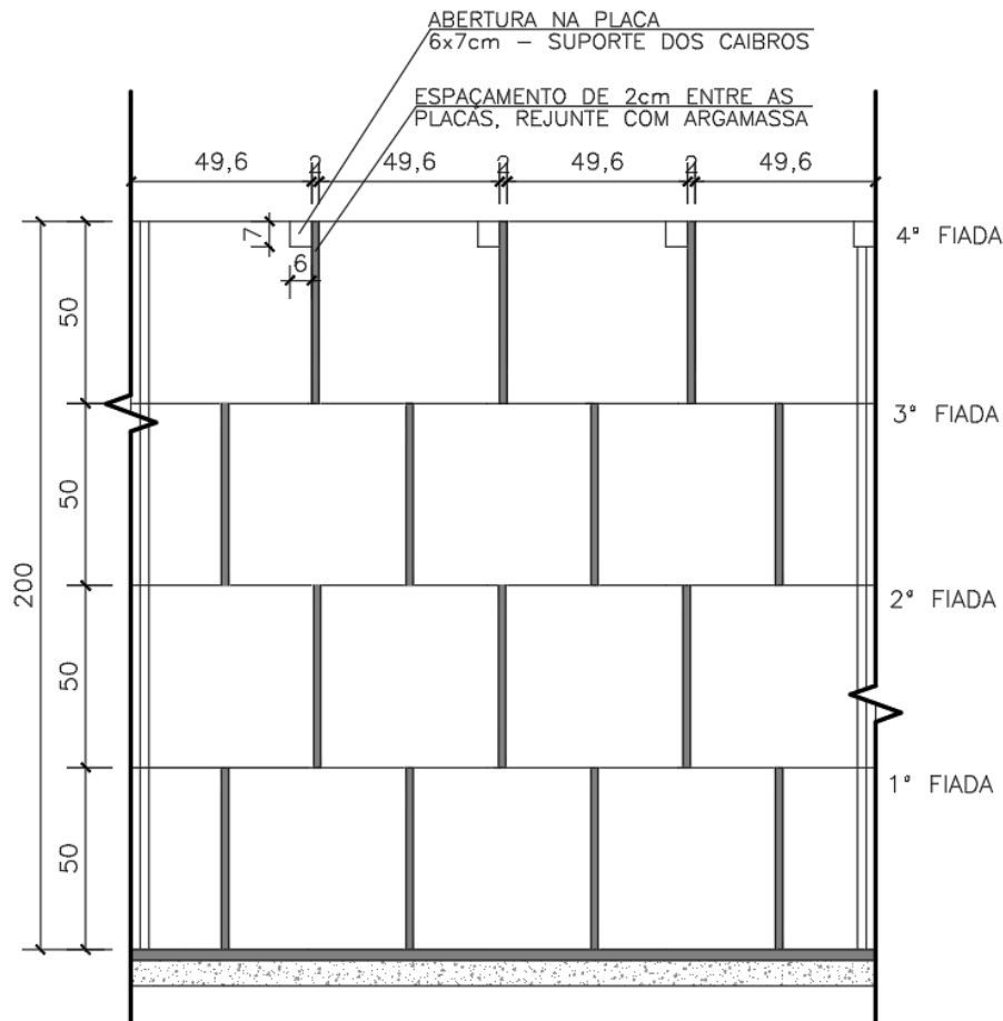
Figura 6.8 – Paginação da parede
