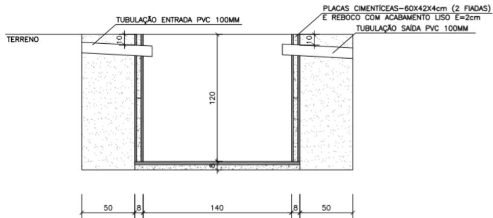
Figura 6.30 - Caixa de Sedimentação com canaleta de entrada – Corte B-B' Fonte: COBRAPE (2021)
