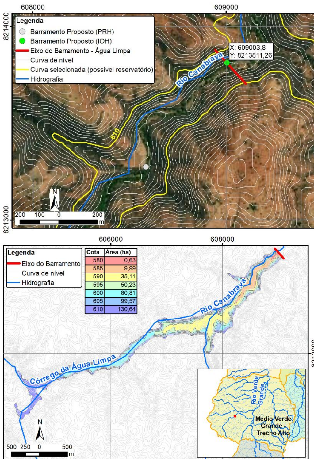
Figura 6.10 - Eixo e Área Alagada do Barramento Água Limpa.
