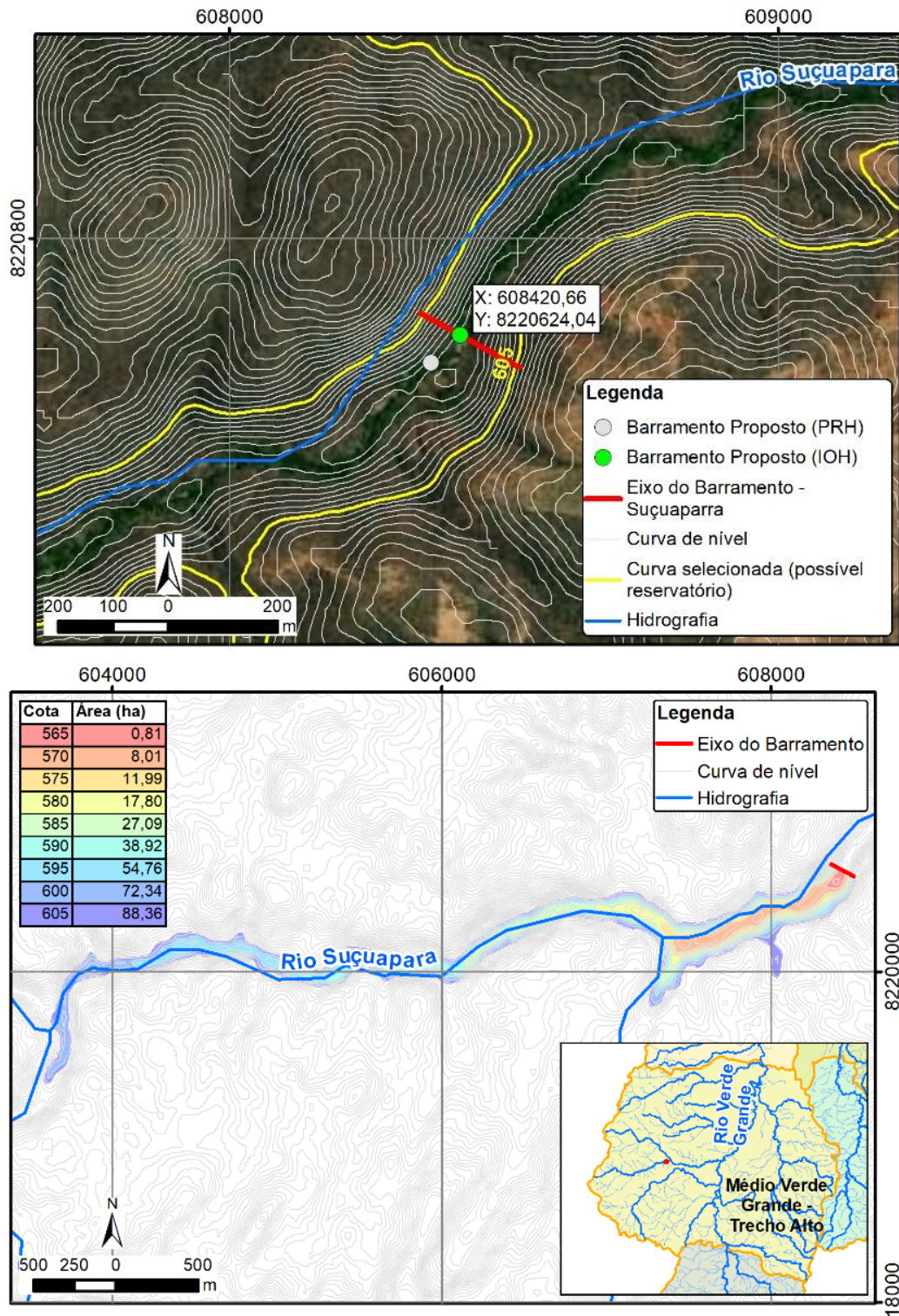
Figura 6.9 - Eixo e Área Alagada do Barramento Suçuaparra.
