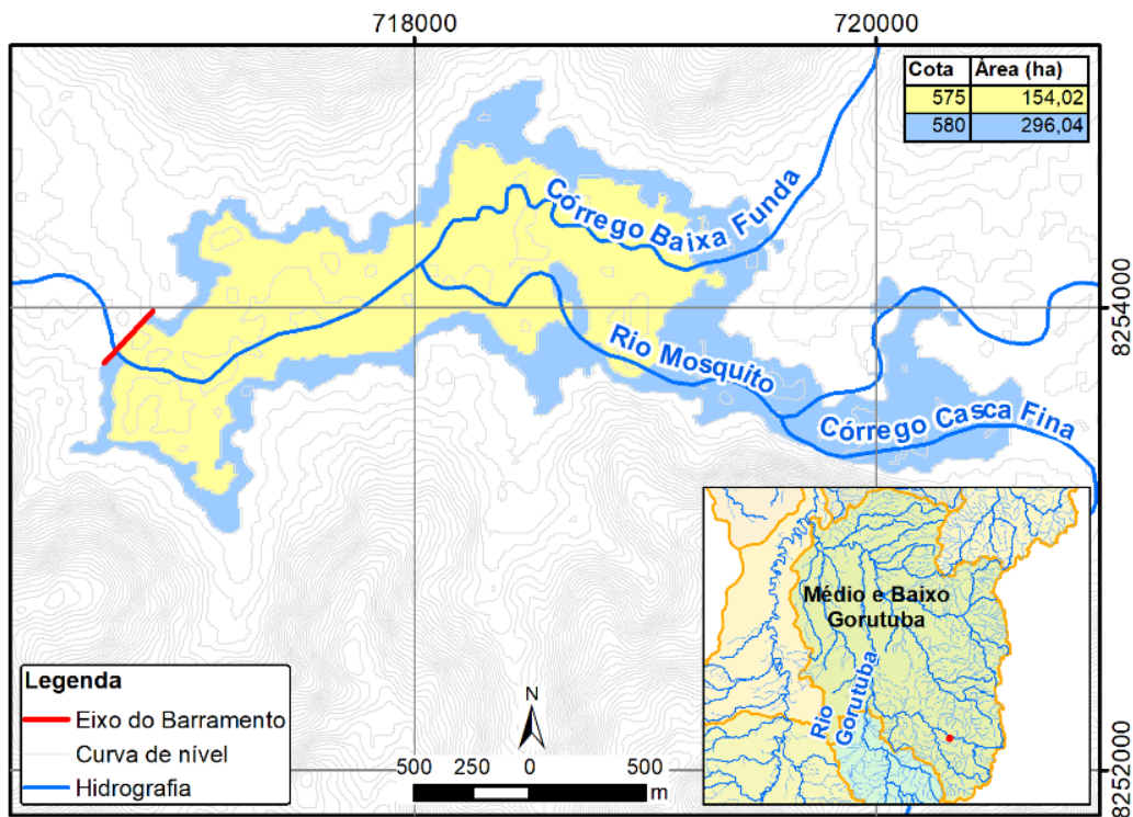
Figura 6.11 - Eixo e Área Alagada do Barramento Cocos.
