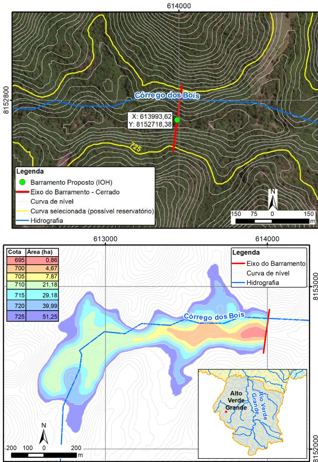
Figura 6.7 - Eixo e Área Alagada do Barramento Cerrado.
