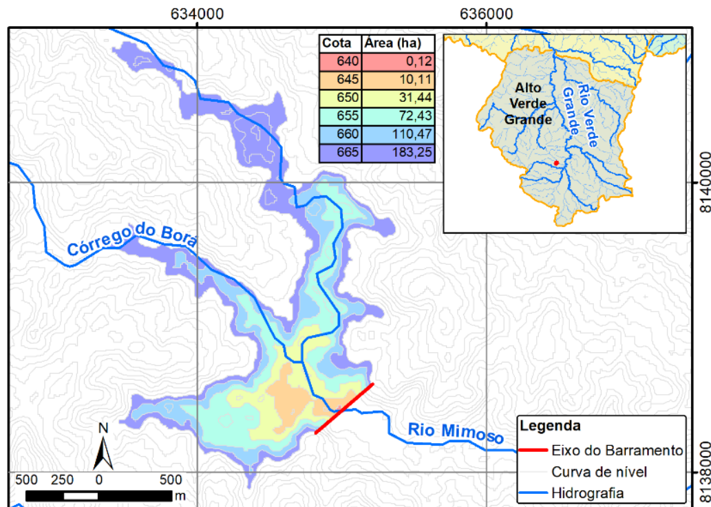
Figura 6.1 - Eixo e Área Alagada do Barramento Peixe
