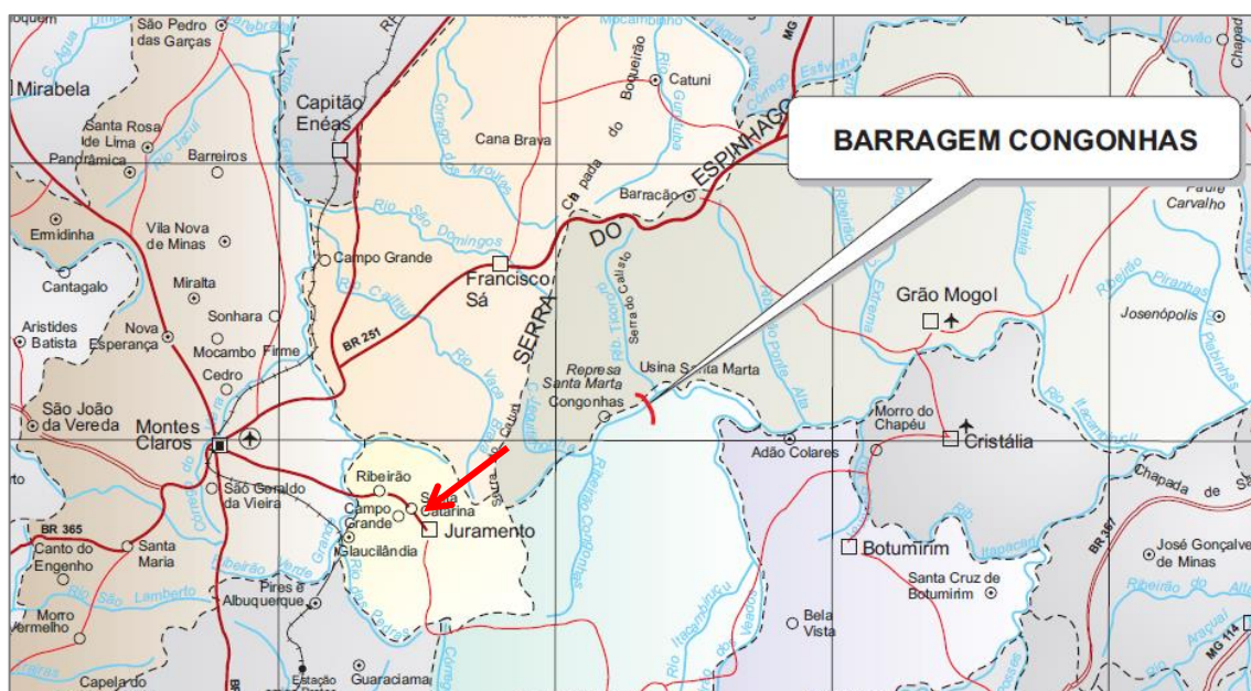
Fonte: Revisão do Projeto Executivo da Barragem Congonhas, 2014.
