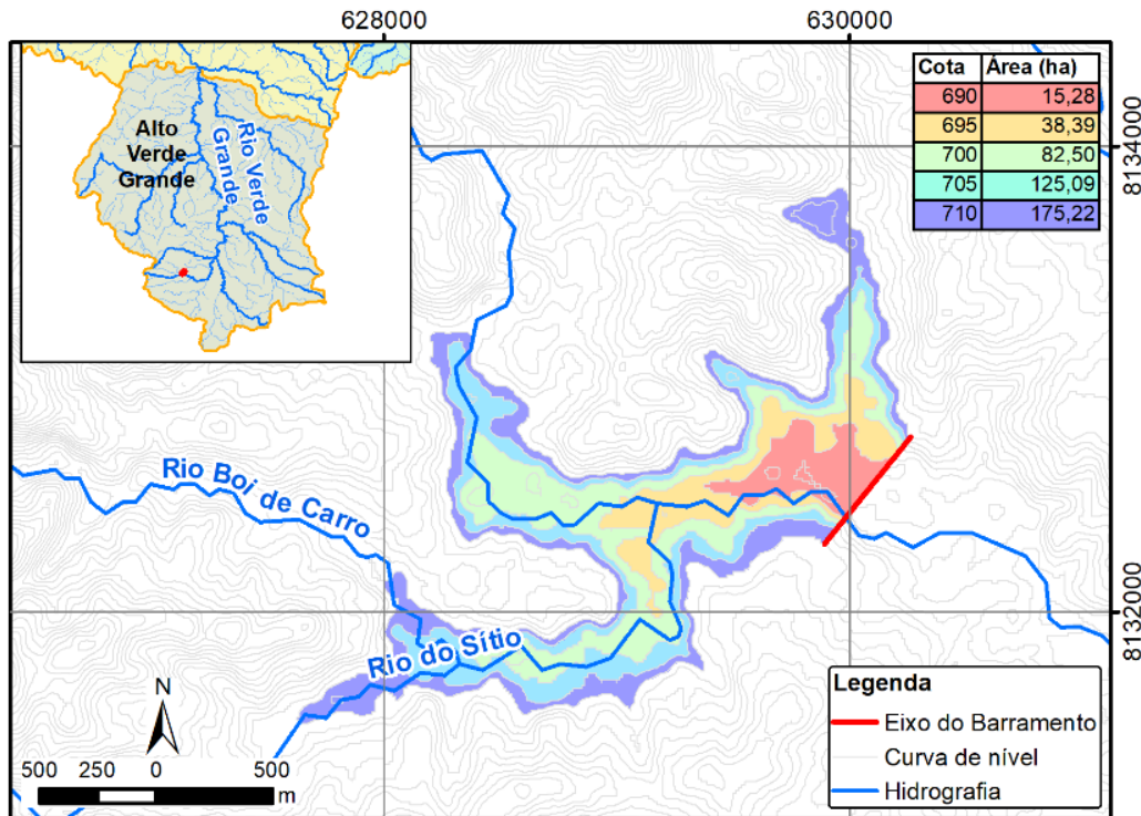
Figura 6.2 - Eixo e Área Alagada do Barramento Sítio.
