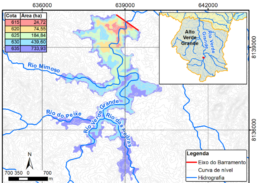
Figura 6.5 - Eixo e Área Alagada do Barramento Verde.
