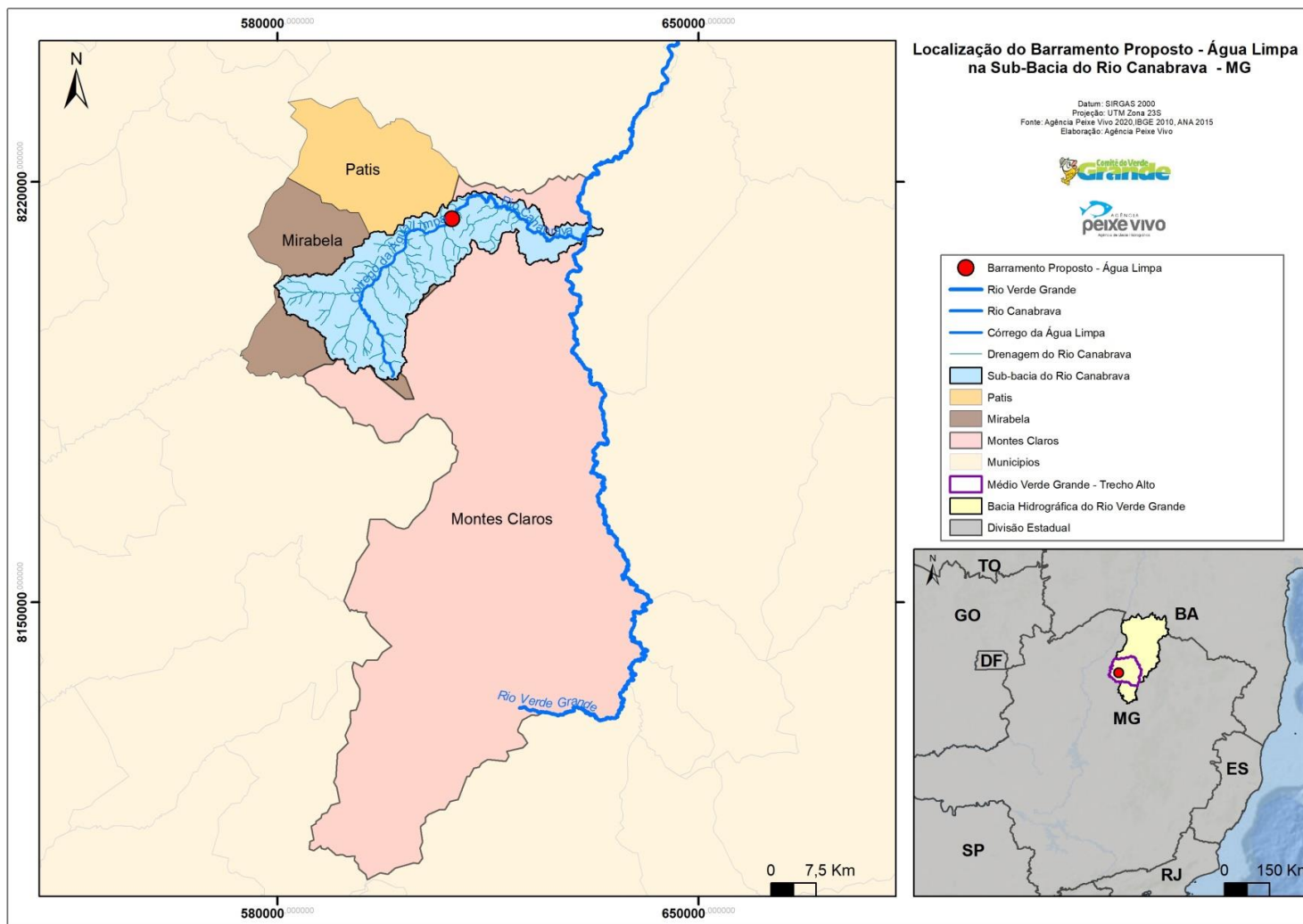
Figura 2: Localização do Barramento - Água Limpa. Fonte: Agência Peixe Vivo, 2020
