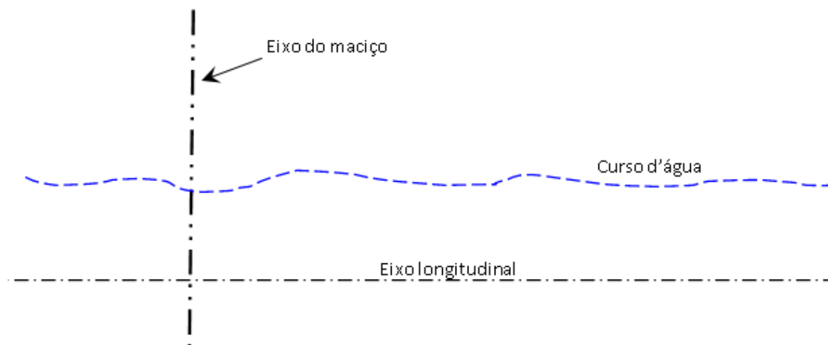
Figura 8: Alinhamento e extensão dos eixos (visão em planta).
