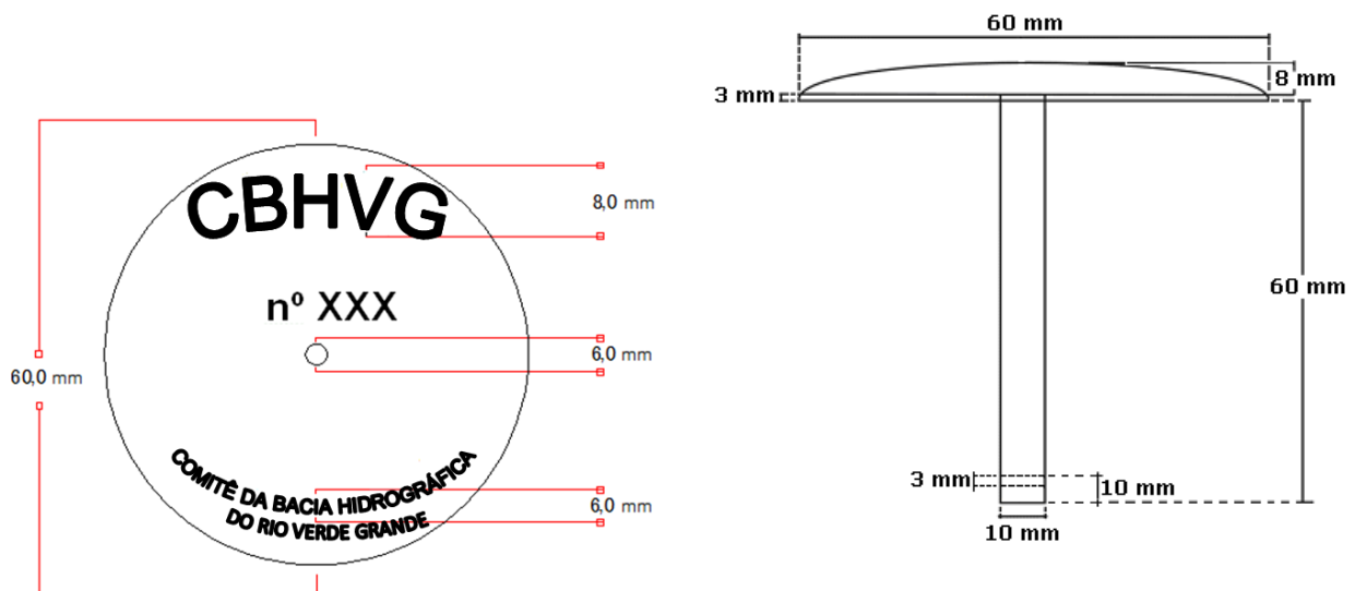
Figura 12: Corte e vista da plaqueta metálica.
