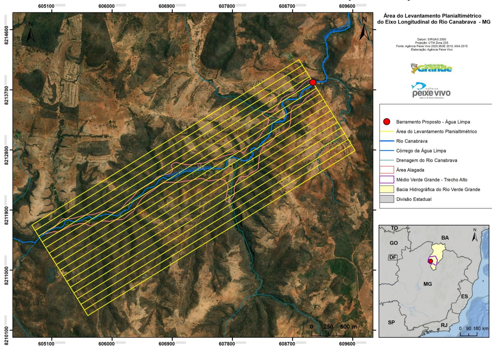
Figura 10: Área do Levantamento Planialtimétrico - Eixo Longitudinal do rio Canabrava. Fonte: Agência Peixe Vivo, 2020.
