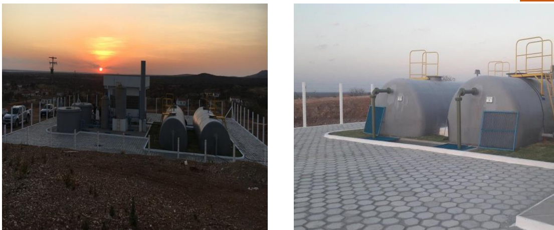
Figura 21 - Acervo fotográfico das obras e serviços de implantação do sistema de abastecimento de água da aldeia Pankará, Itacuruba - PE (Fonte: TANTO Expresso, 2018).
