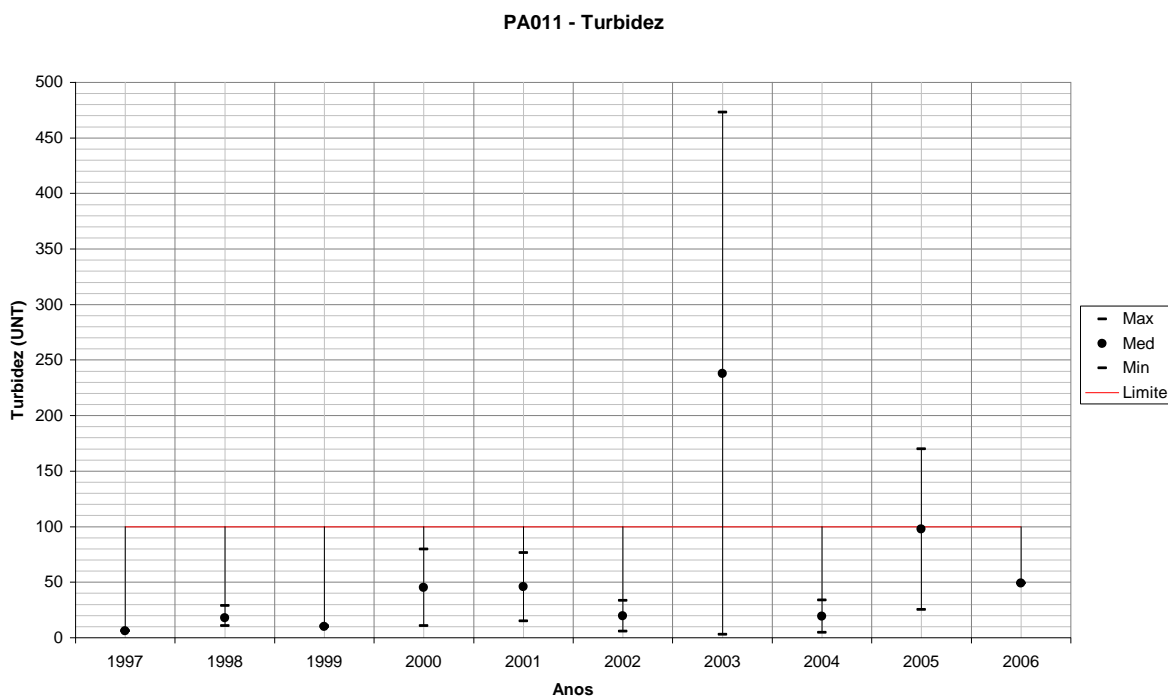
Figura 227 – Variação de Turbidez para PA011 em relação ao período úmido de cada ano monitorado.
