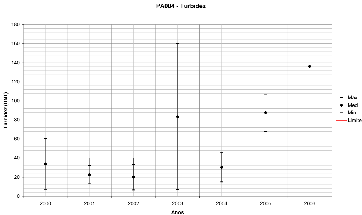
Figura 157 – Variação de Turbidez para PA004 em relação ao período úmido de cada ano monitorado.
