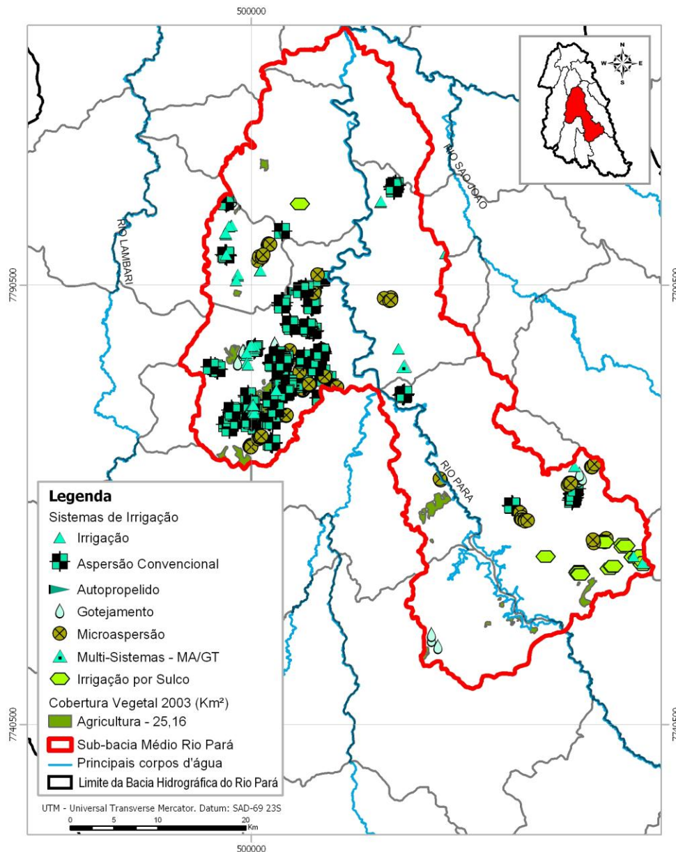
Figura 79 – Pontos de captação para irrigação na Sub-bacia Médio Rio Pará
