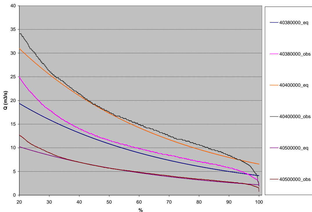
Figura 57 – Ajuste da equação exponencial às curvas de permanência da região homogênea IV.
