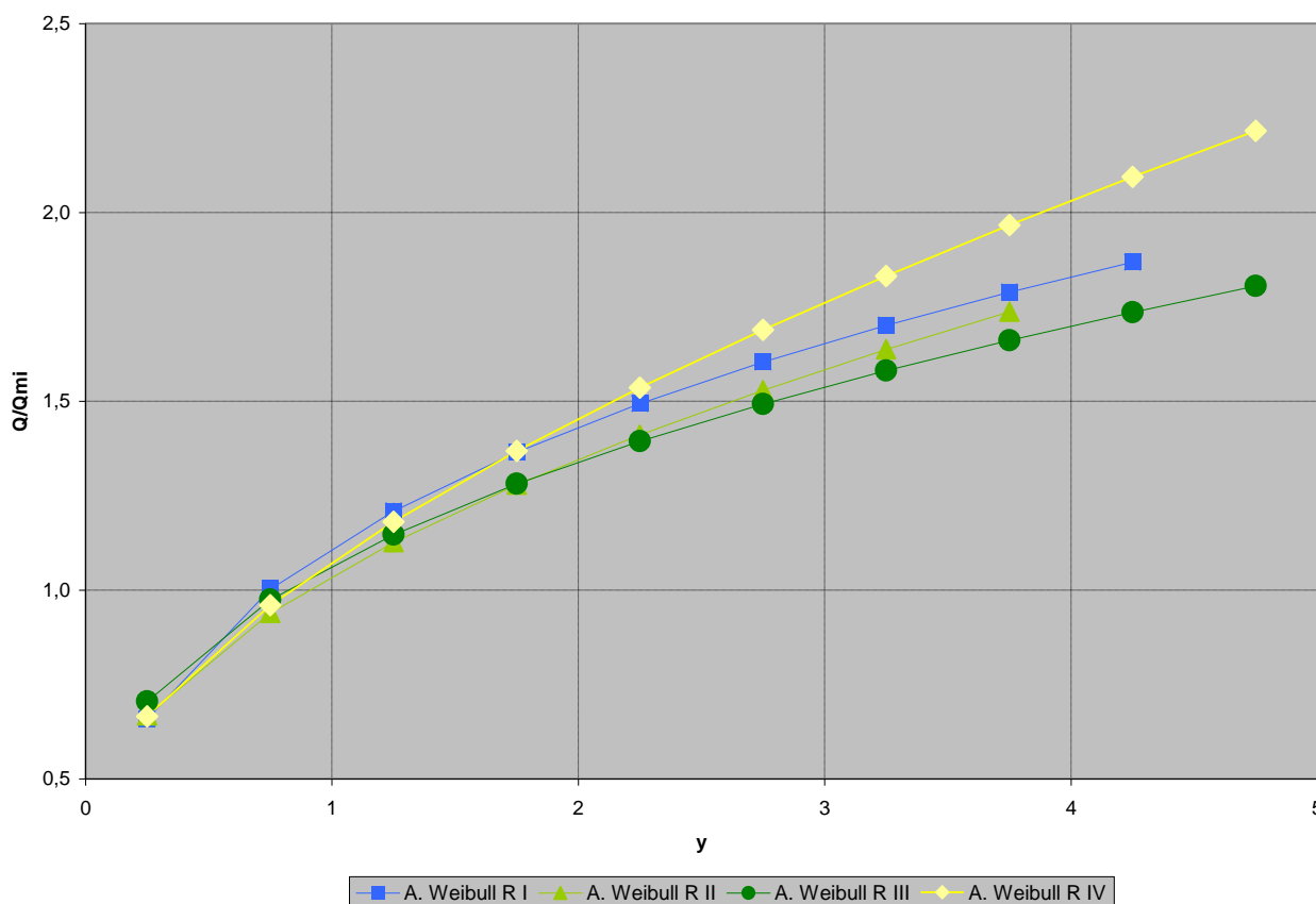
Figura 49 – Ajuste da distribuição estatística de Weibull aos pontos médios das regiões homogêneas.
