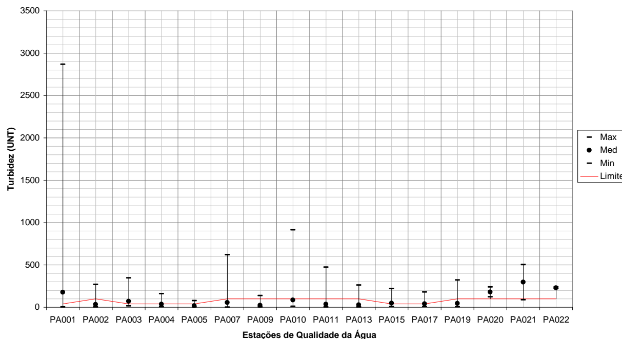
Figura 120 – Variação de Turbidez para todas as estações de qualidade da água em relação a todo o período monitorado.
