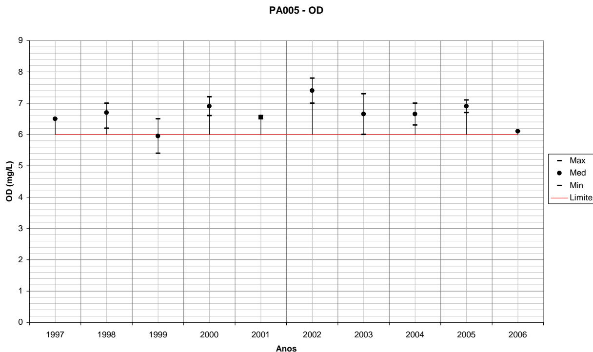
Figura 173 – Variação de OD para PA005 em relação ao período úmido de cada ano monitorado.
