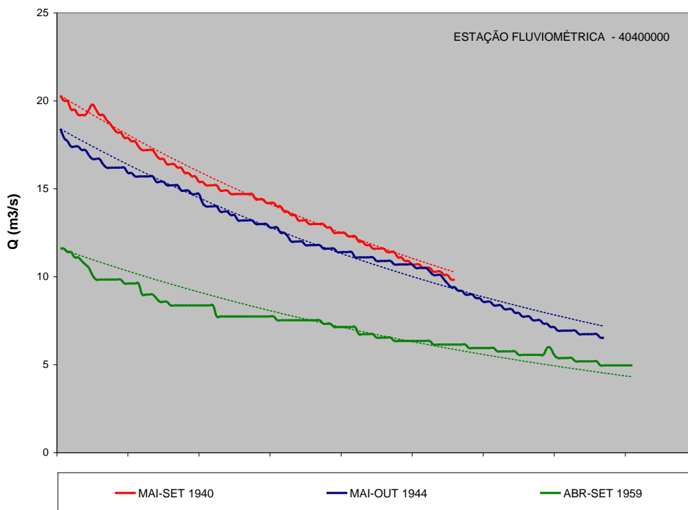
Figura 61 – Ajuste da curva de depleção teórica para a região homogênea IV de vazões mínimas
