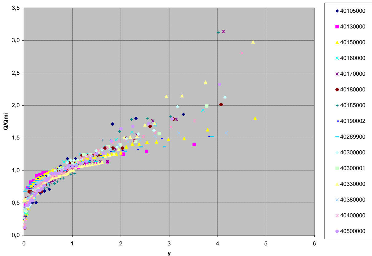
Figura 47 – Curvas individuais de probabilidade para vazões mínimas
