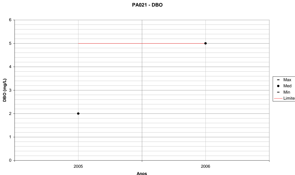
Figura 254 – Variação de DBO para PA021 em todos os anos monitorados.
