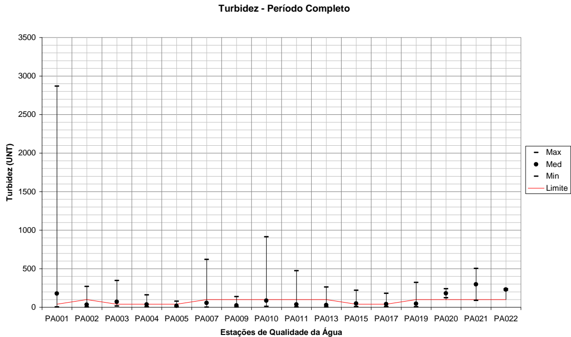
Figura 244 – Variação de Turbidez para todas as estações de qualidade da água em relação a todo o período monitorado.
