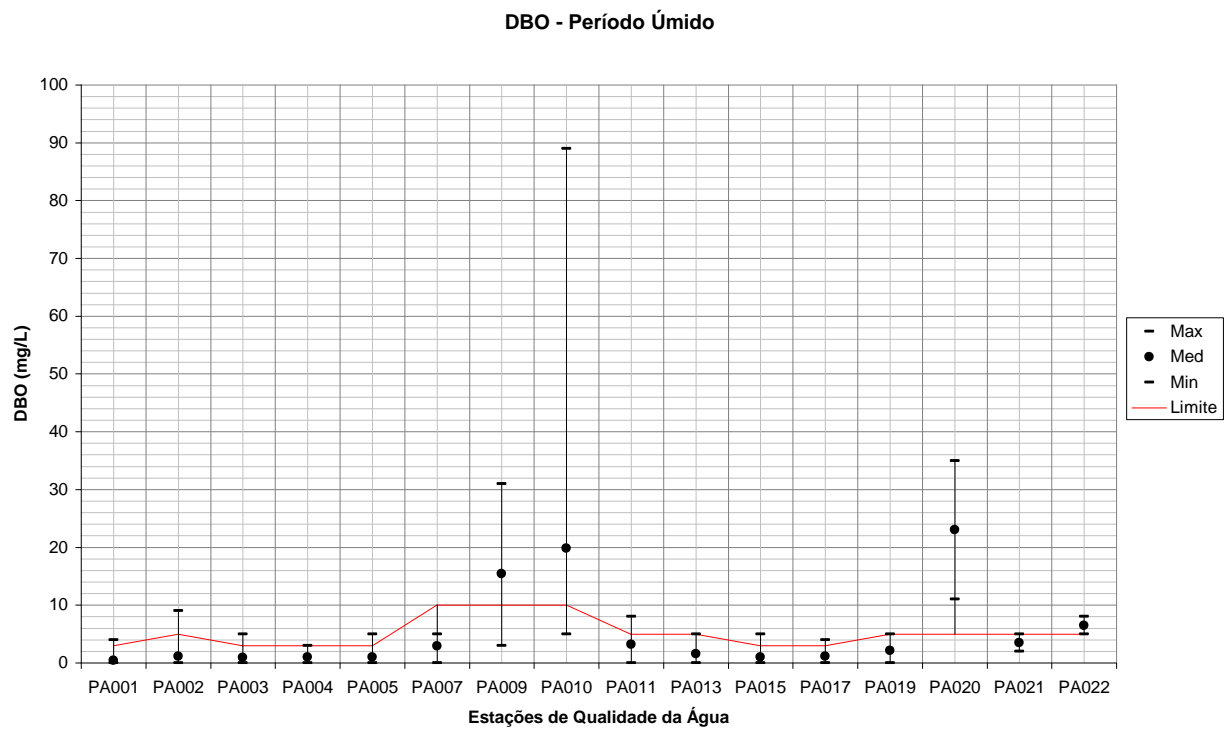
Figura 104 – Variação de DBO para todas as estações de qualidade da água em relação a todo o período úmido.
