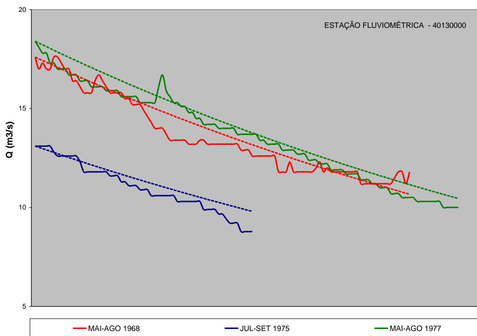
Figura 58 – Ajuste da curva de depleção teórica para a região homogênea I de vazões mínimas
