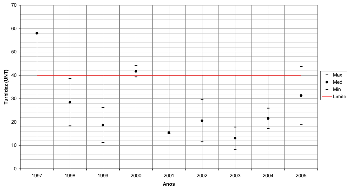
Figura 248 – Variação de Turbidez para PA015 em relação ao período seco de cada ano monitorado.
