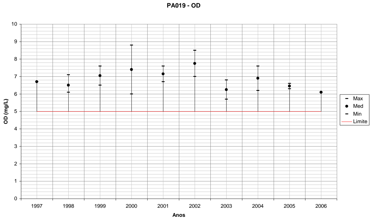
Figura 293 – Variação de OD para PA019 em relação ao período úmido de cada ano monitorado.
