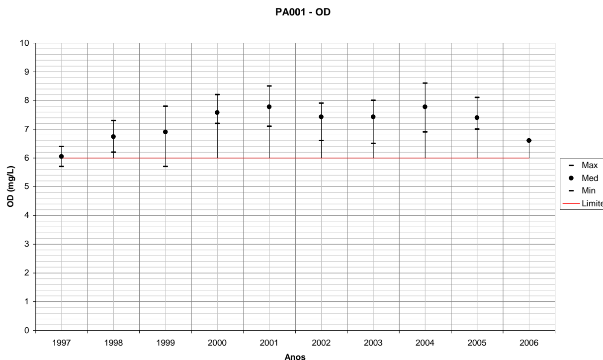
Figura 109 – Variação de OD para PA001 em todos os anos monitorados.
