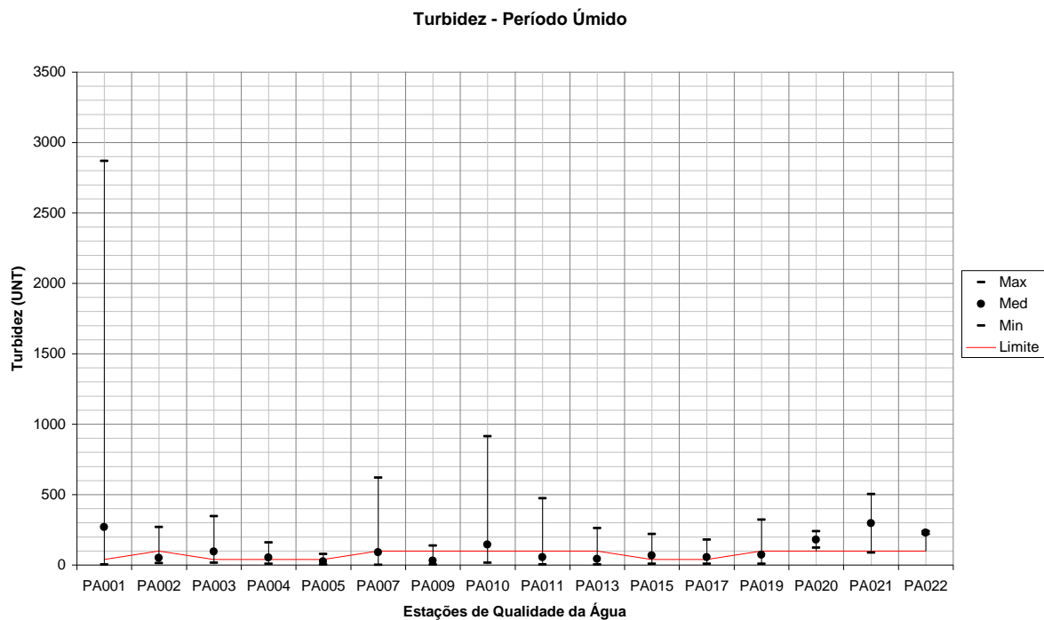
Figura 273 – Variação da Turbidez para todas as estações de qualidade da água em relação a todo o período úmido.
