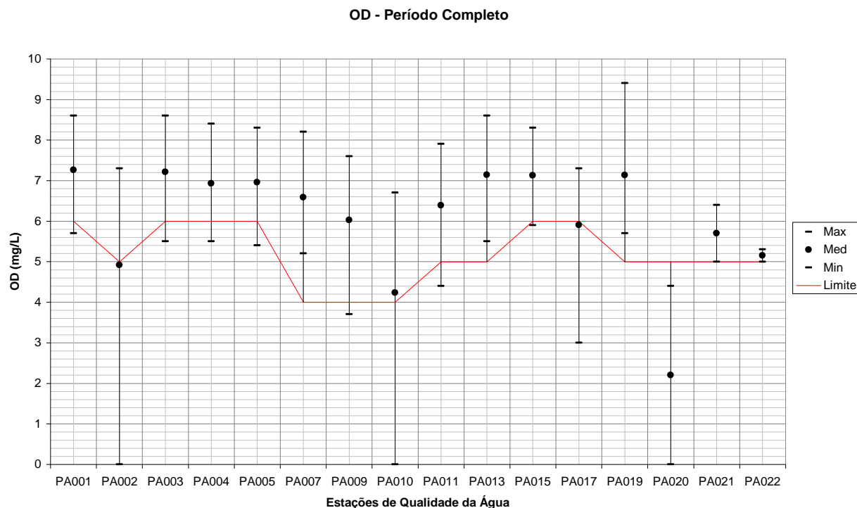
Figura 260 – Variação de OD para todas as estações de qualidade da água em relação a todo o período monitorado.
