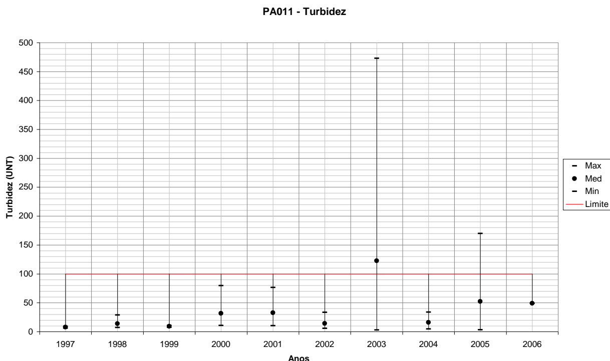
Figura 221 – Variação de Turbidez para PA011 em todos os anos monitorados.
