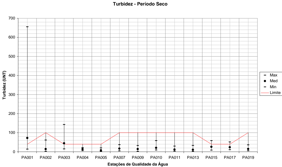
Figura 153 – Variação de Turbidez para todas as estações de qualidade da água em relação a todo o período seco.
