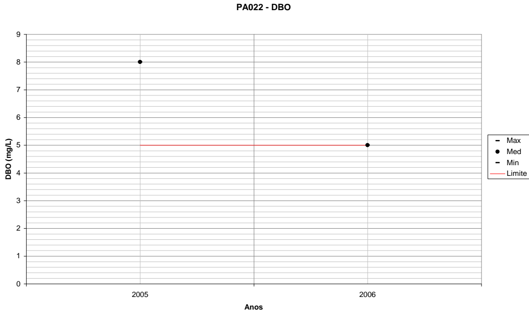
Figura 235 – Variação de DBO para PA022 em relação ao período úmido de cada ano monitorado. Fonte: IGAM. Processamento TESE Tecnologia em Sistemas Espaciais Ltda.
