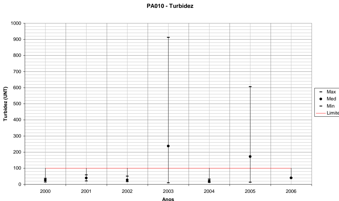
Figura 196 – Variação de Turbidez para PA010 em todos os anos monitorados.
