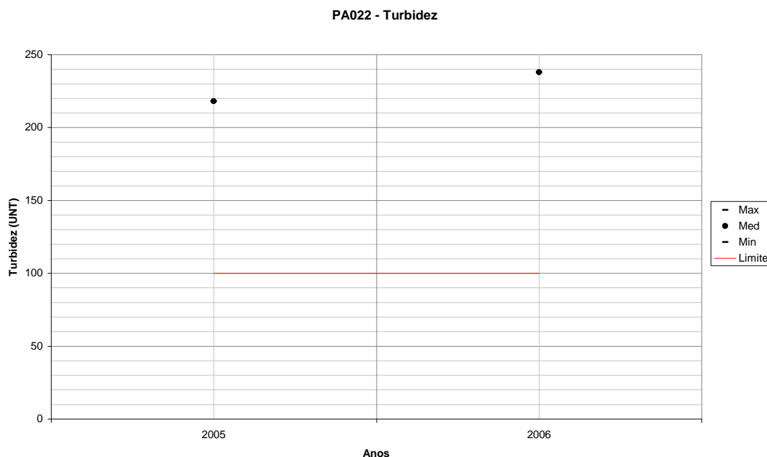
Figura 246 – Variação de Turbidez para PA022 em todos os anos monitorados. Fonte: IGAM. Processamento TESE Tecnologia em Sistemas Espaciais Ltda.
