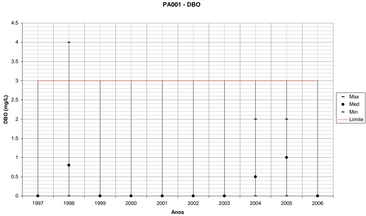
Figura 97 – Variação de DBO para PA001 em todos os anos monitorados.
