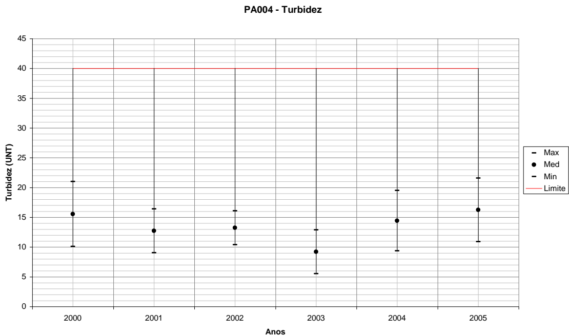
Figura 154 – Variação de Turbidez para PA004 em relação ao período seco de cada ano monitorado.
