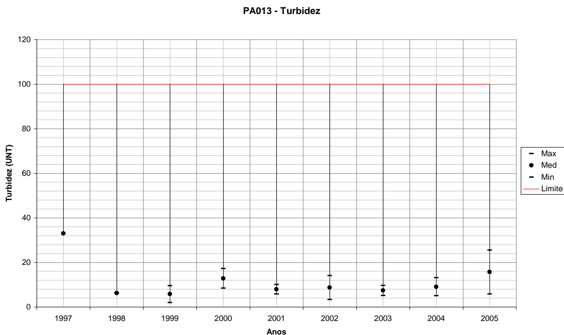
Figura 298 – Variação de Turbidez para PA013 em relação ao período seco de cada ano monitorado.
