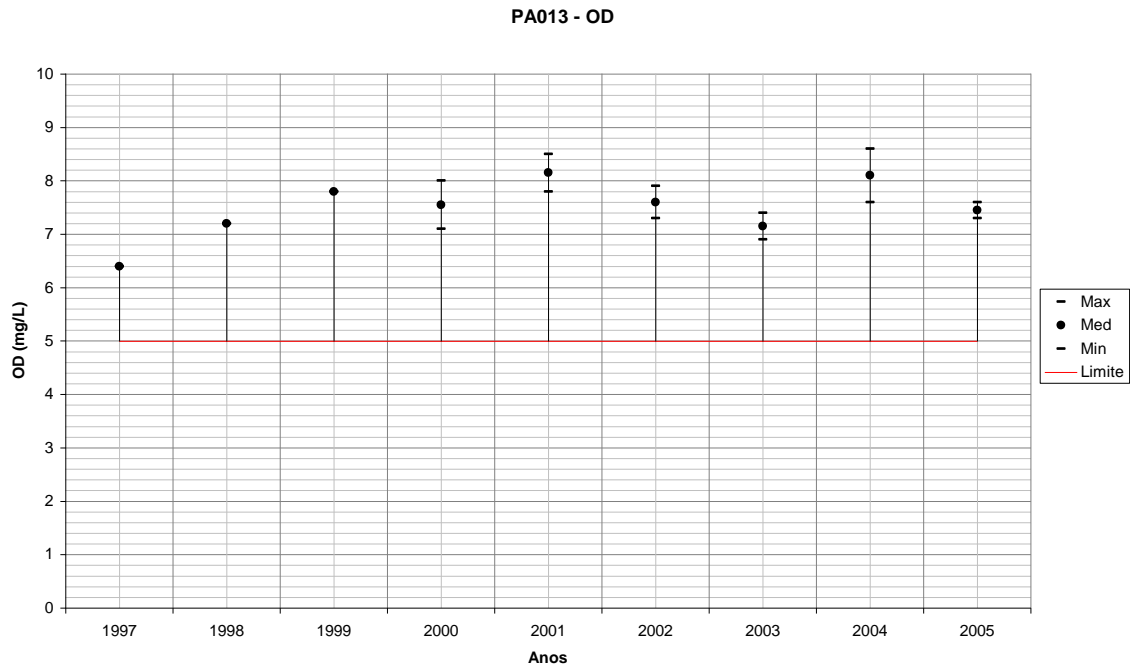
Figura 289 – Variação de OD para PA013 em relação ao período seco de cada ano monitorado. Fonte: IGAM. Processamento TESE Tecnologia em Sistemas Espaciais Ltda.
