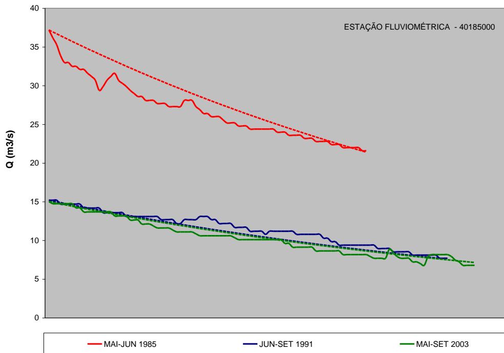
Figura 59 – Ajuste da curva de depleção teórica para a região homogênea II de vazões mínimas Fonte: Processamento de informações pela TESE Tecnologia em Sistemas Espaciais Ltda.
