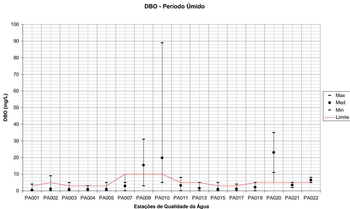
Figura 282 – Variação de DBO para todas as estações de qualidade da água em relação a todo o período úmido.
