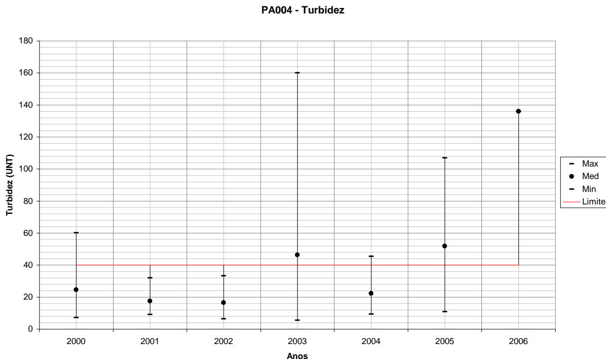
Figura 151 – Variação de Turbidez para PA004 em todos os anos monitorados.
