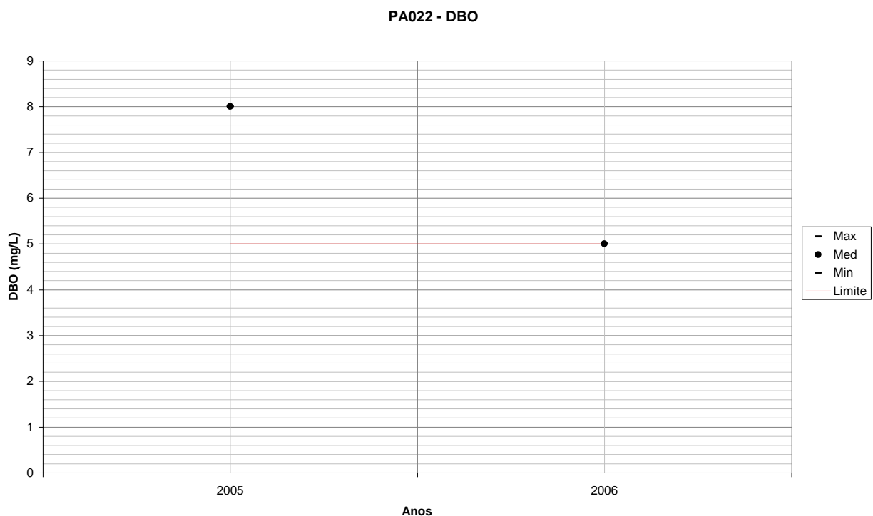
Figura 230 – Variação de DBO para PA022 em todos os anos monitorados.
