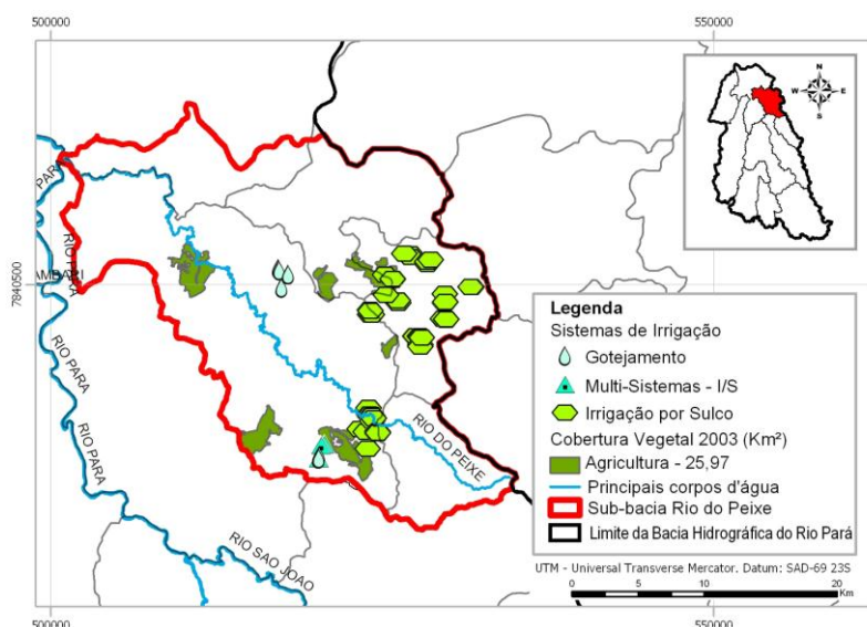
Figura 83 – Pontos de captação para irrigação na Sub-bacia Rio do Peixe
