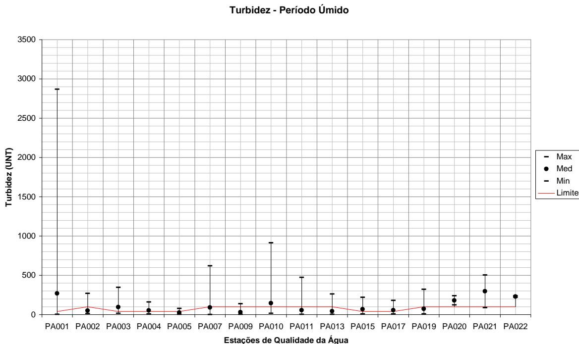
Figura 249 – Variação da Turbidez para todas as estações de qualidade da água em relação a todo o período úmido.
