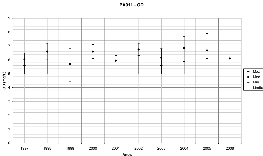
Figura 212 – Variação de OD para PA011 em todos os anos monitorados.
