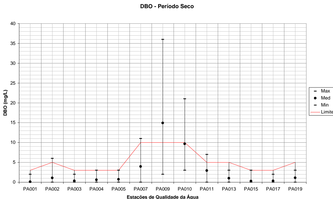
Figura 255 – Variação de DBO para todas as estações de qualidade da água em relação a todo o período seco.
