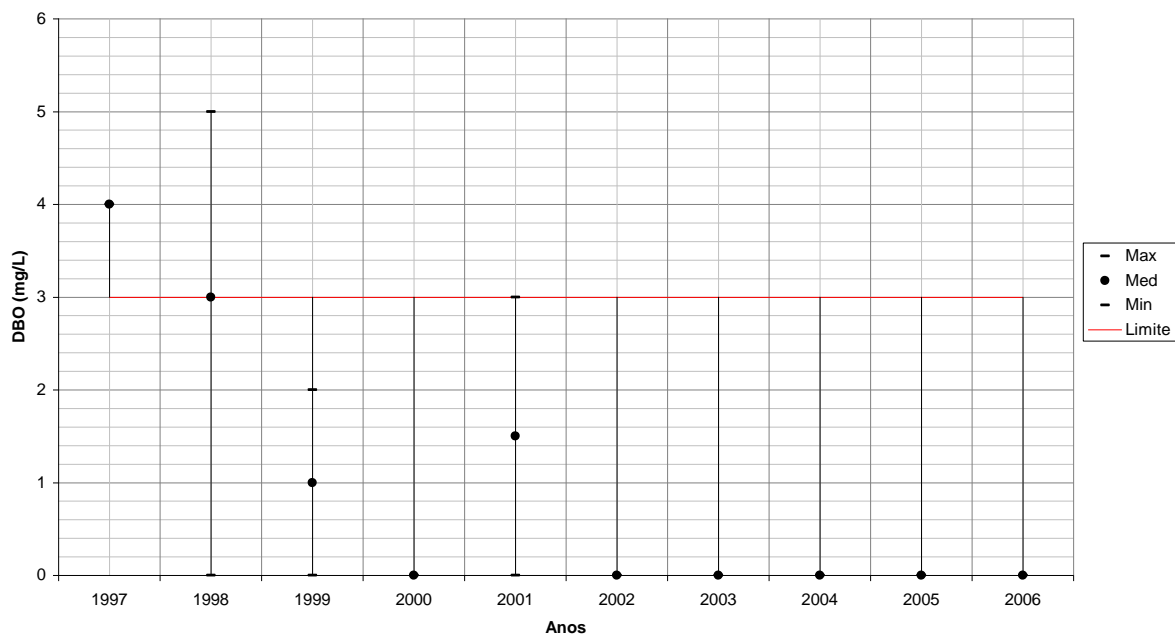
Figura 107 – Variação de DBO para PA003 em relação ao período úmido de cada ano monitorado. Fonte: IGAM. Processamento TESE Tecnologia em Sistemas Espaciais Ltda.
