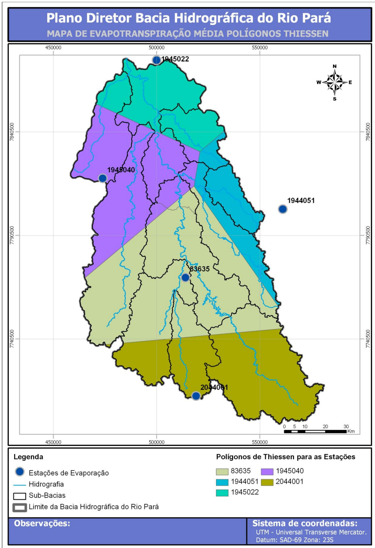
Figura 63 – Polígonos de Thiessen para o cálculo da evapotranspiração média na Bacia Hidrográfica do Rio Pará
