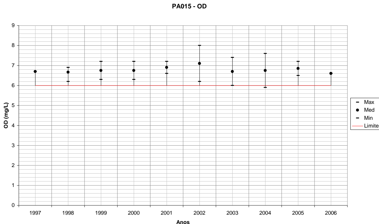
Figura 242 – Variação de OD para PA015 em relação ao período úmido de cada ano monitorado. Fonte: IGAM. Processamento TESE Tecnologia em Sistemas Espaciais Ltda.
