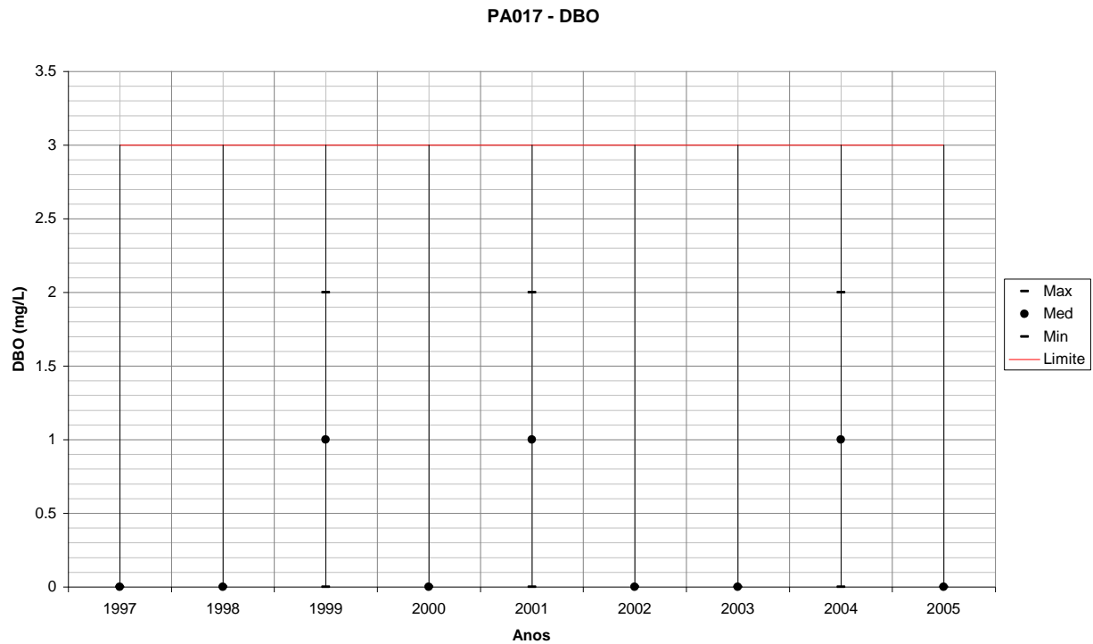
Figura 256 – Variação de DBO para PA017 em relação ao período seco de cada ano monitorado.
