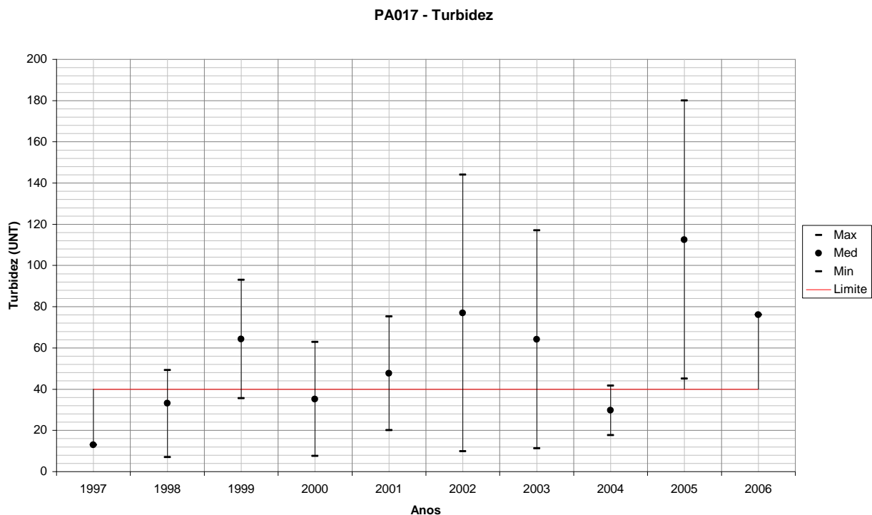
Figura 274 – Variação de Turbidez para PA017 em relação ao período úmido de cada ano monitorado.
