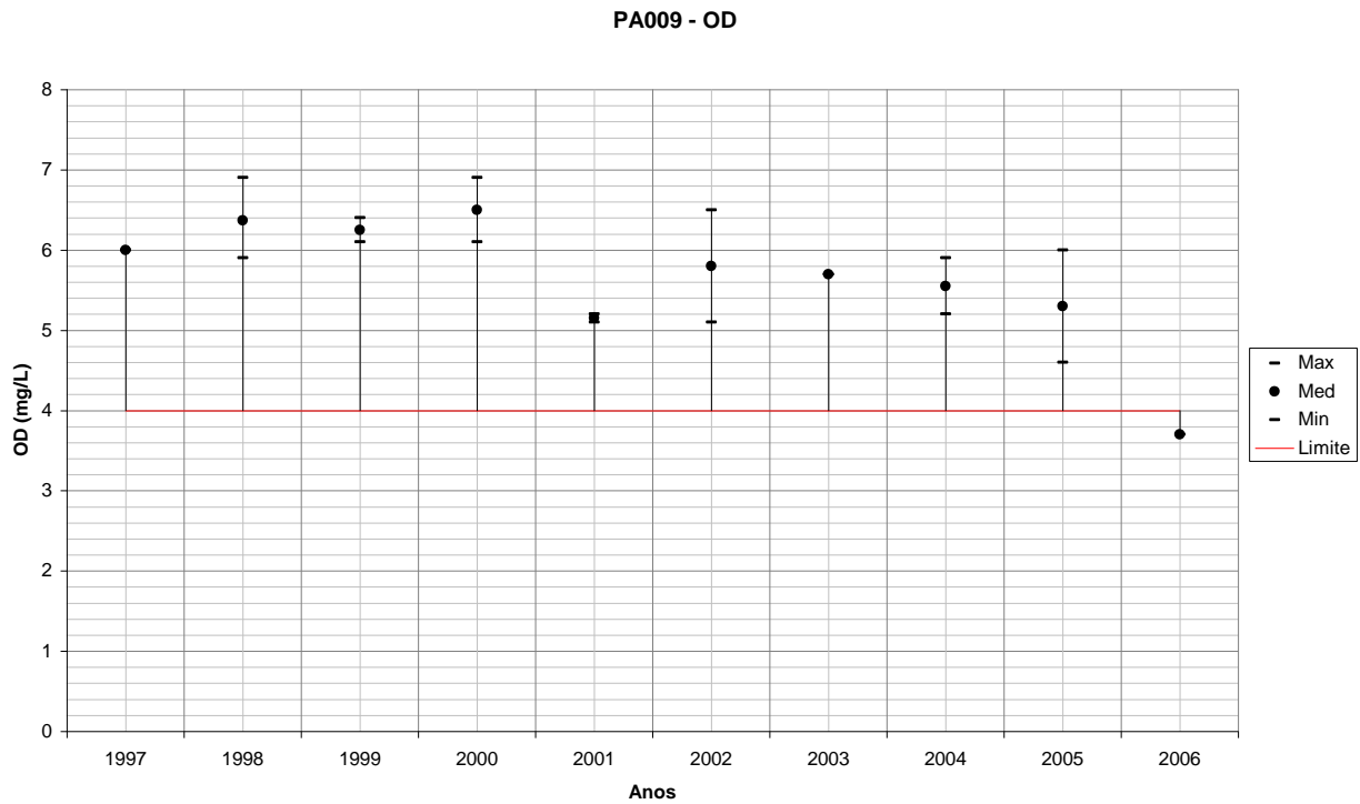
Figura 217 – Variação de OD para PA009 em relação ao período úmido de cada ano monitorado.
