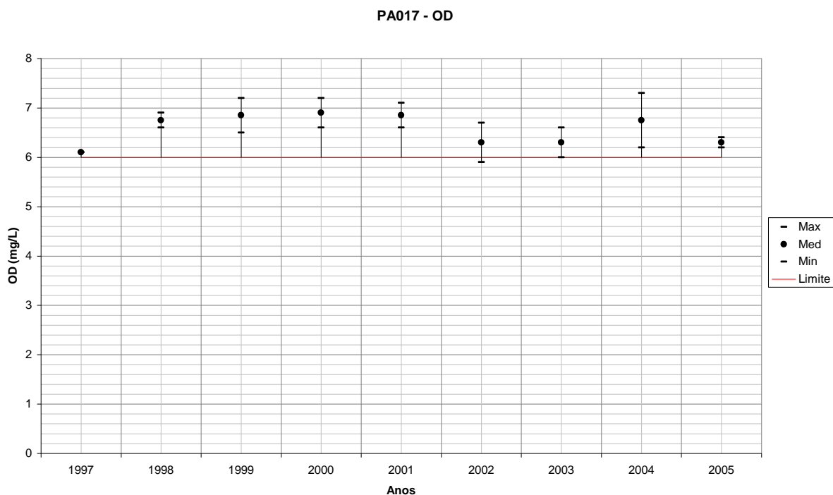
Figura 264 – Variação de OD para PA017 em relação ao período seco de cada ano monitorado.
