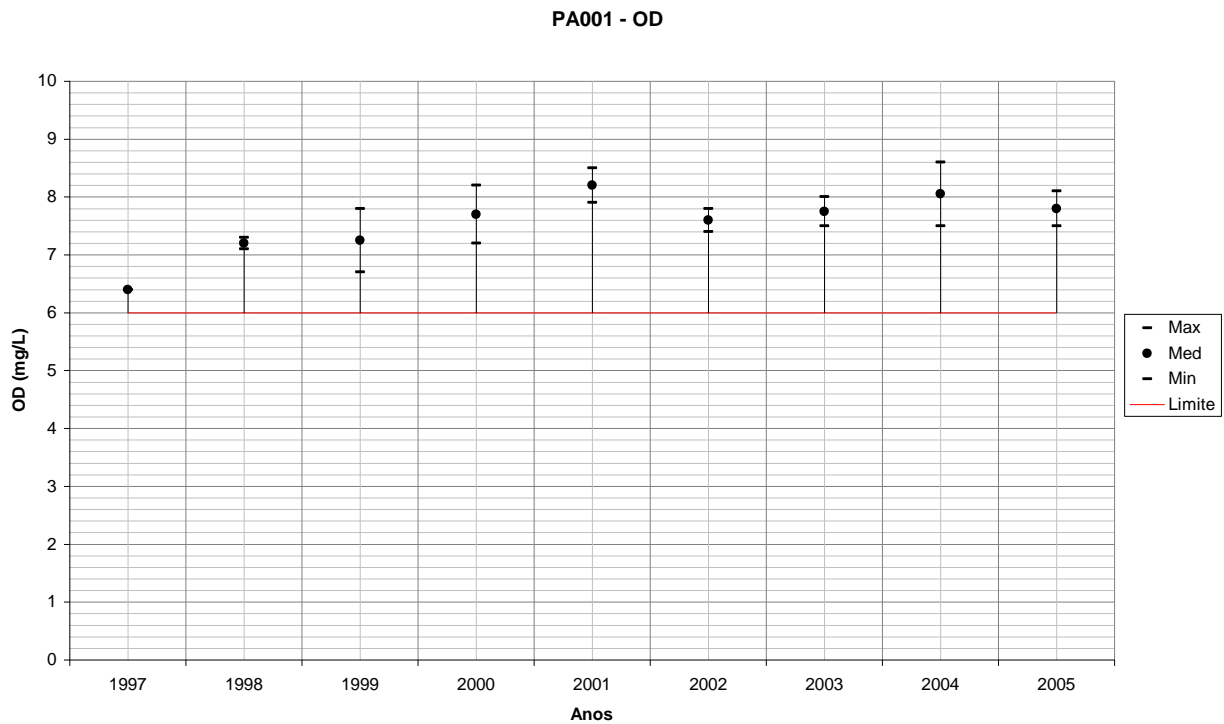
Figura 113 – Variação de OD para PA001 em relação ao período seco de cada ano monitorado.
