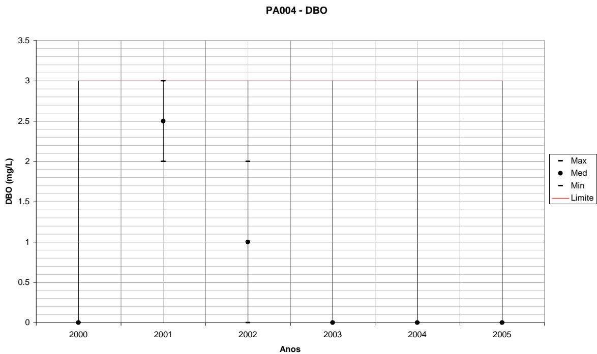
Figura 136 – Variação de DBO para PA004 em relação ao período seco de cada ano monitorado.
