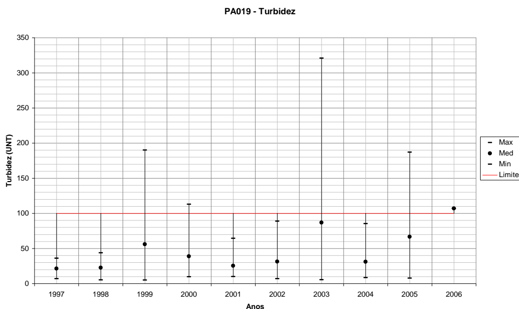
Figura 296 – Variação de Turbidez para PA019 em todos os anos monitorados.
