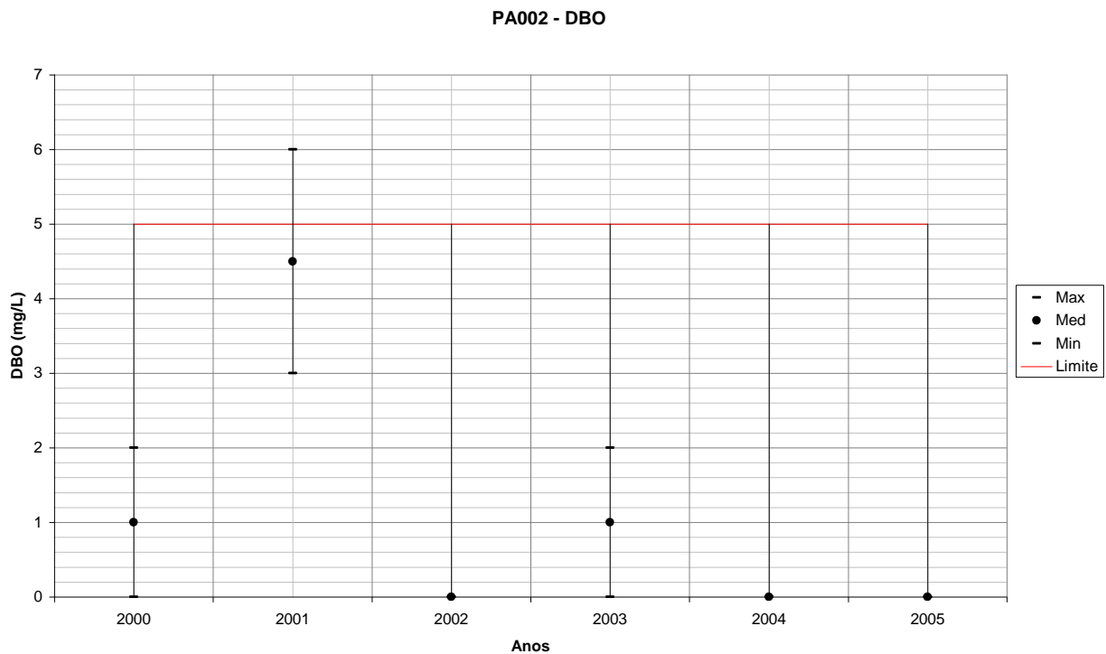
Figura 102 – Variação de DBO para PA002 em relação ao período seco de cada ano monitorado.
