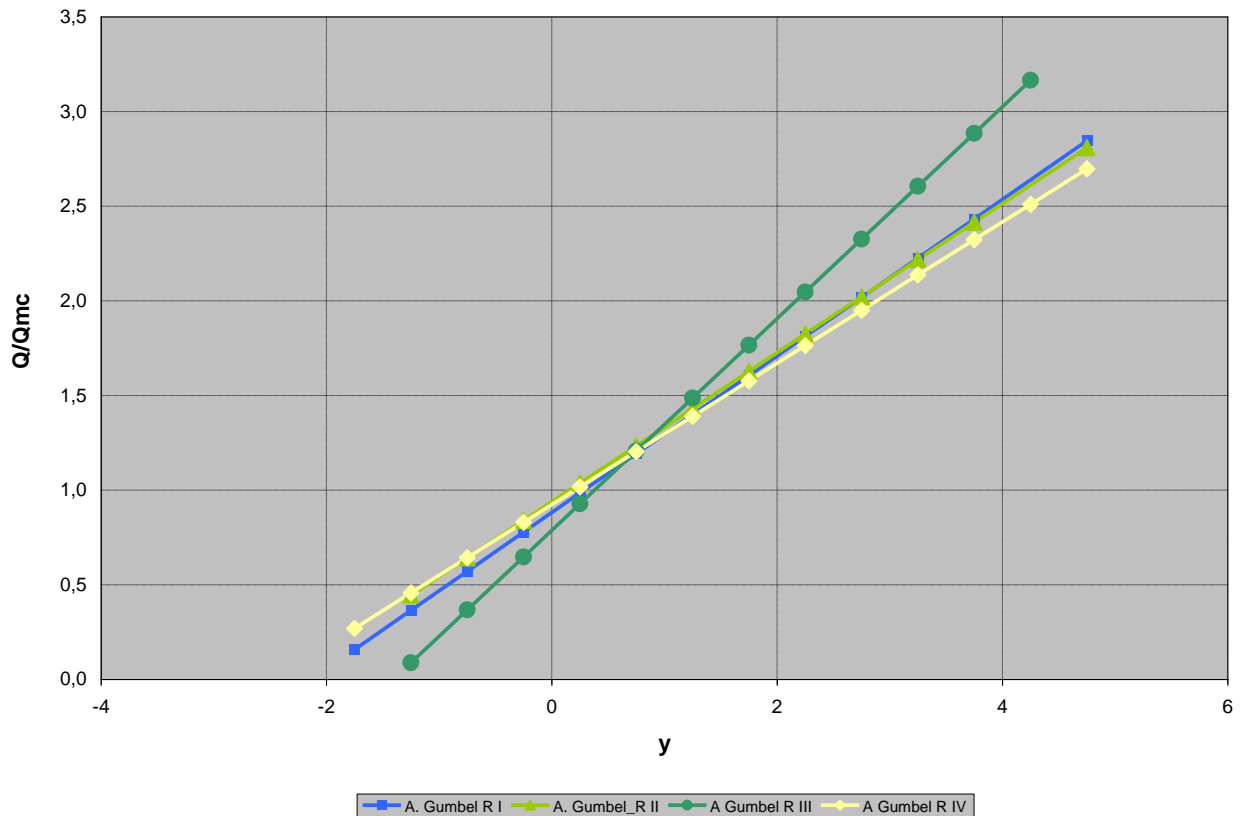
Figura 52 – Ajuste da distribuição estatística de Gumbel aos pontos médios das regiões homogêneas para as vazões máximas.
