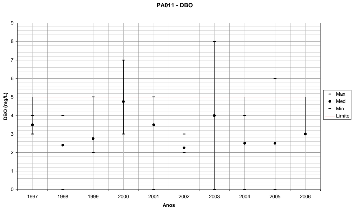
Figura 203 – Variação de DBO para PA011 em todos os anos monitorados.
