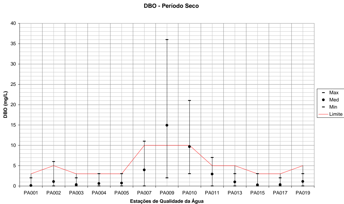
Figura 162 – Variação de DBO para todas as estações de qualidade da água em relação a todo o período seco.
