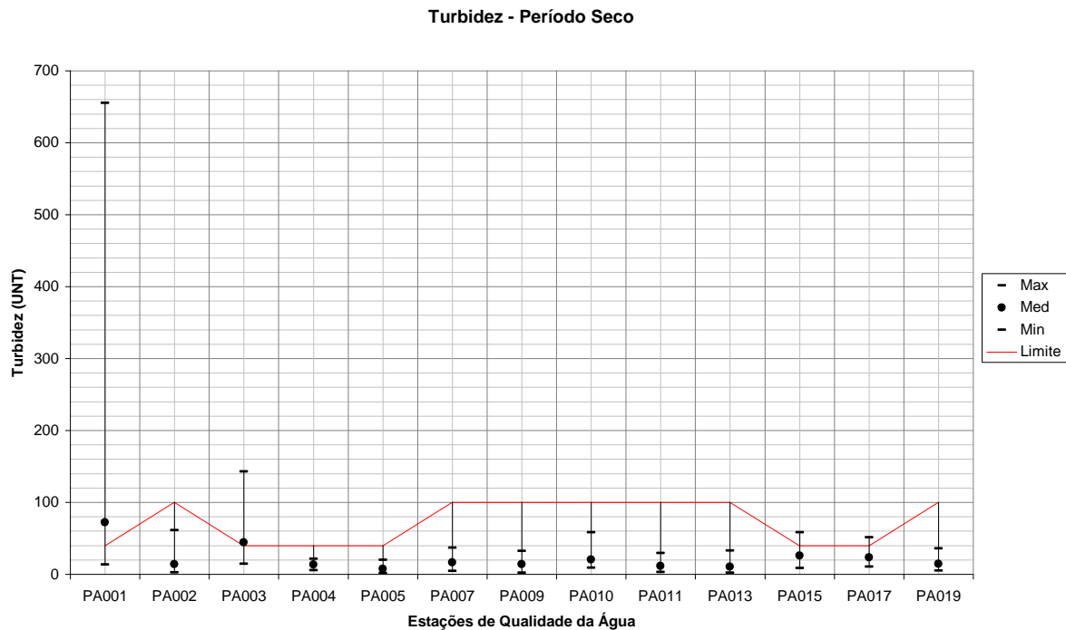
Figura 222 – Variação de Turbidez para todas as estações de qualidade da água em relação a todo o período seco.
