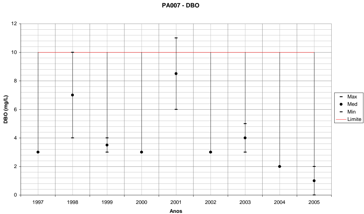
Figura 137 – Variação de DBO para PA007 em relação ao período seco de cada ano monitorado.
