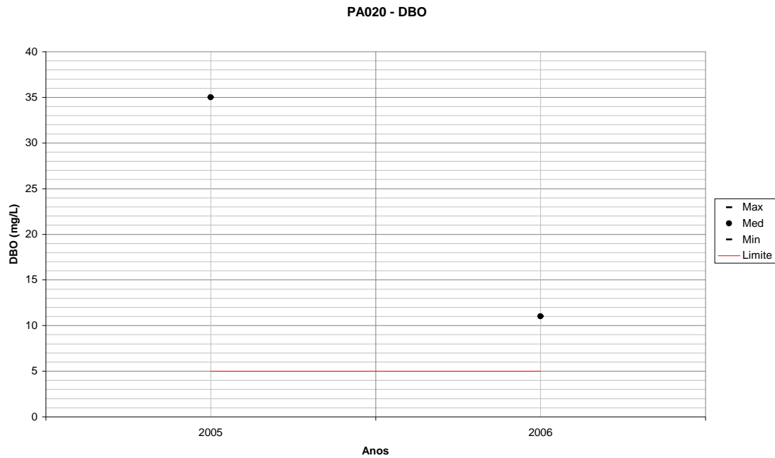
Figura 166 – Variação de DBO para PA020 em relação ao período úmido de cada ano monitorado. Fonte: IGAM. Processamento TESE Tecnologia em Sistemas Espaciais Ltda.
