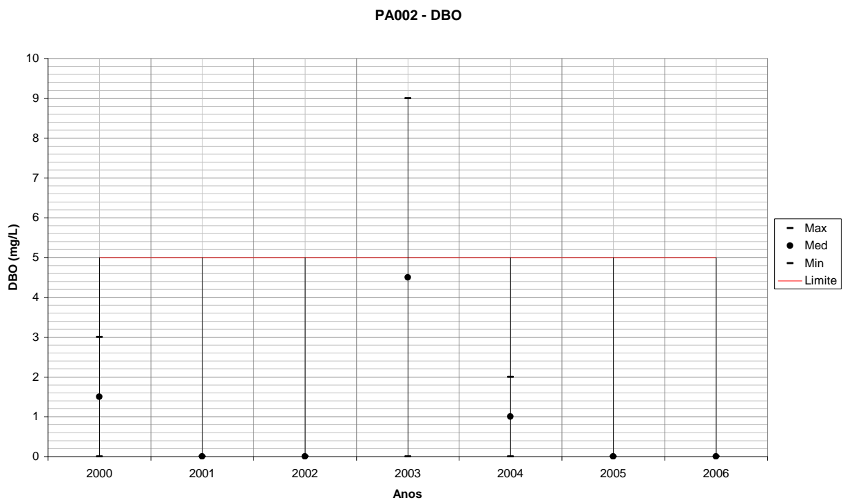
Figura 106 – Variação de DBO para PA002 em relação ao período úmido de cada ano monitorado.
