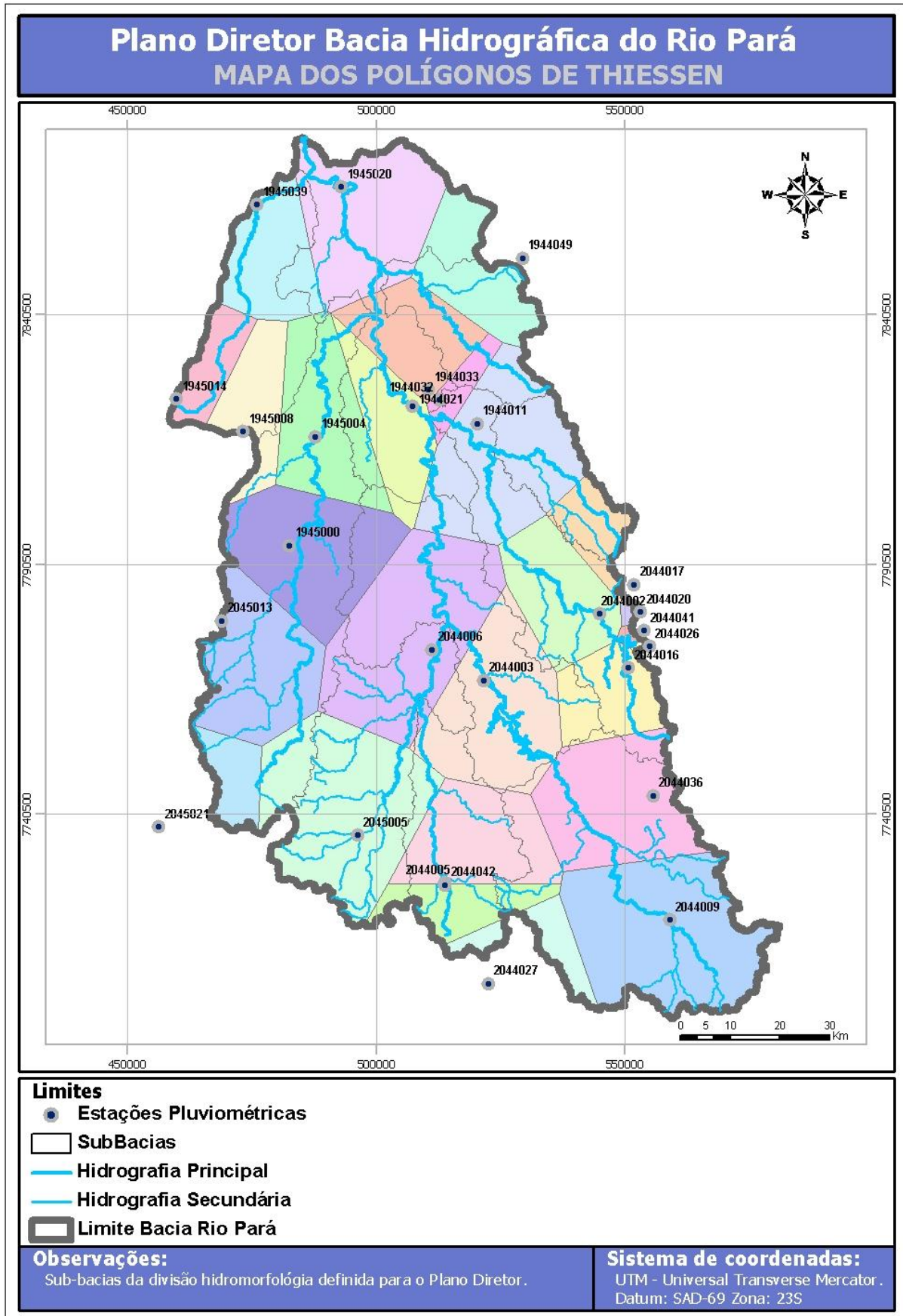
Figura 42 – Polígonos de Thiessen para o cálculo de precipitação na Bacia Hidrográfica do Rio Pará
