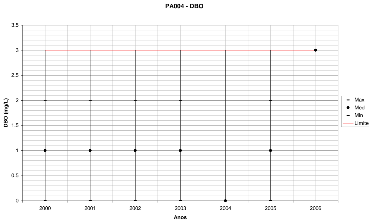
Figura 139 – Variação de DBO para PA004 em relação ao período úmido de cada ano monitorado.
