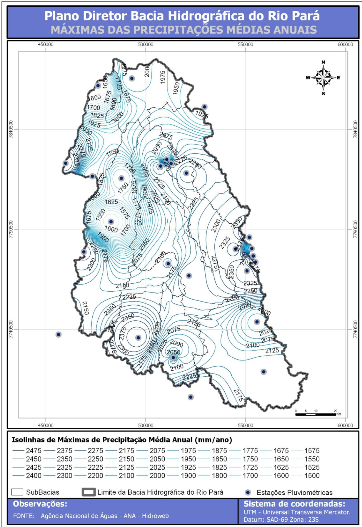
Figura 40 – Isoietas da precipitação média anual máxima
