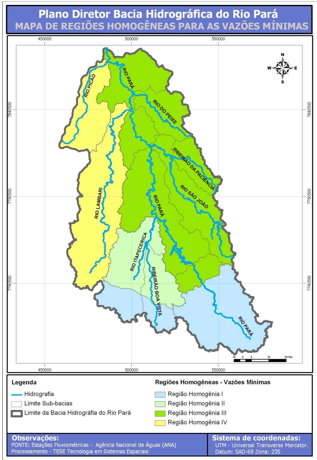
Figura 48 – Regiões homogêneas para as vazões mínimas.
