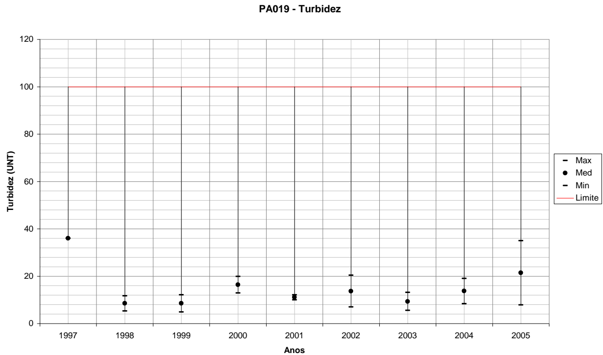
Figura 299 – Variação de Turbidez para PA019 em relação ao período seco de cada ano monitorado.
