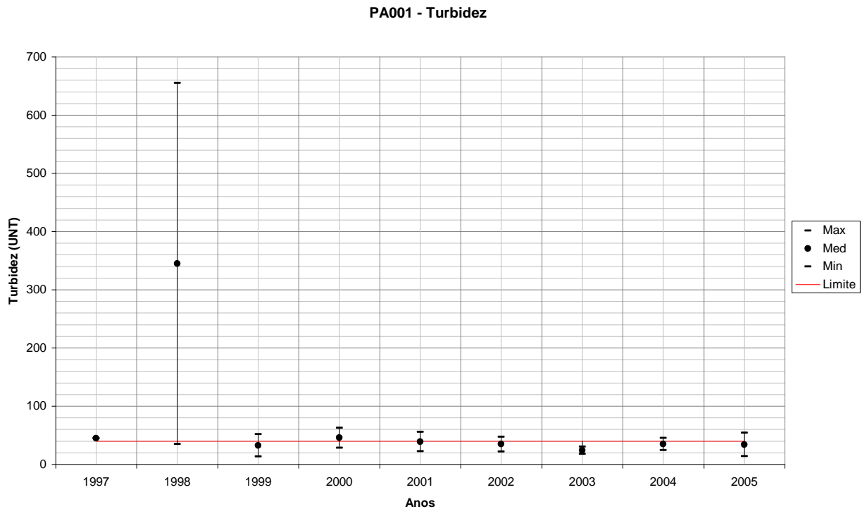
Figura 125 – Variação de Turbidez para PA001 em relação ao período seco de cada ano monitorado.
