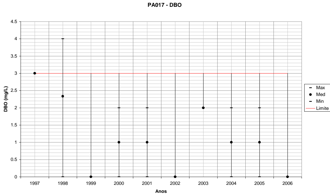
Figura 258 – Variação de DBO para PA017 em relação ao período úmido de cada ano monitorado. Fonte: IGAM. Processamento TESE Tecnologia em Sistemas Espaciais Ltda.
