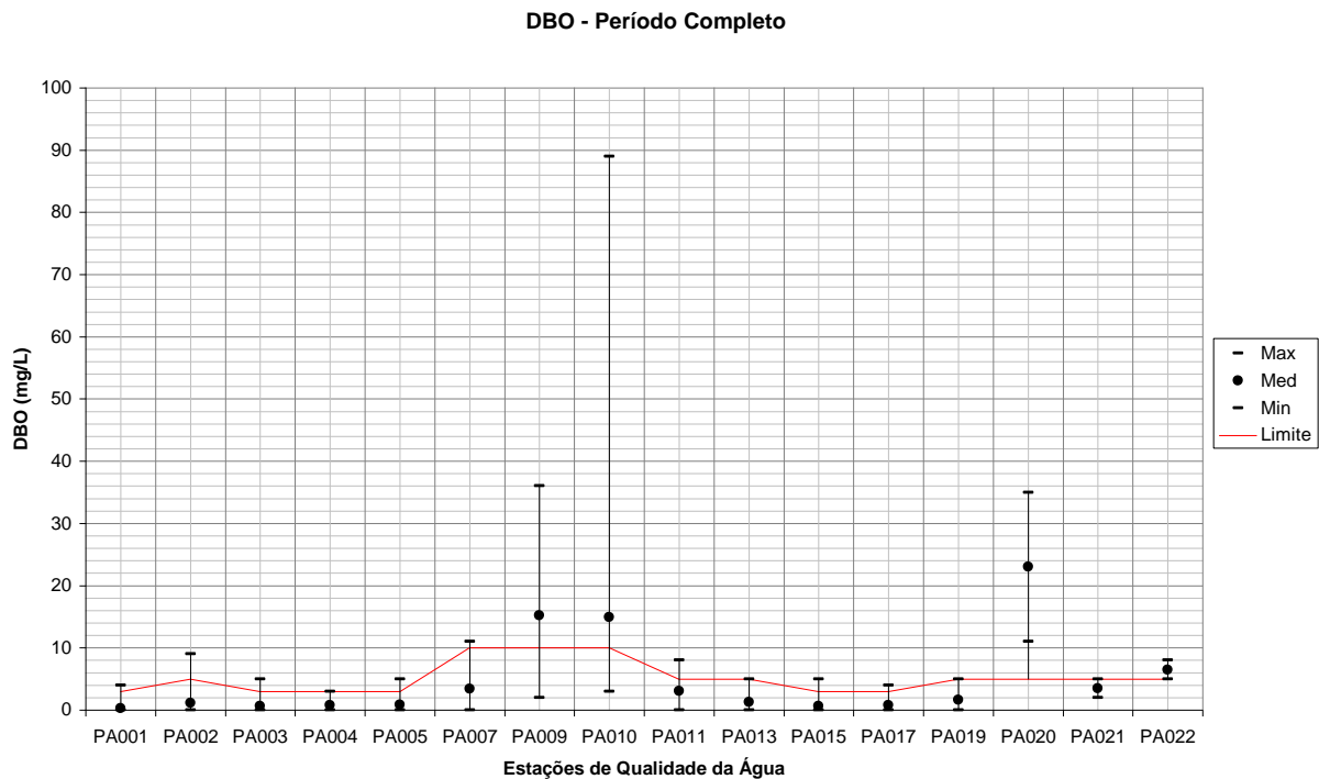
Figura 132 – Variação de DBO para todas as estações de qualidade da água em relação a todo o período monitorado.
