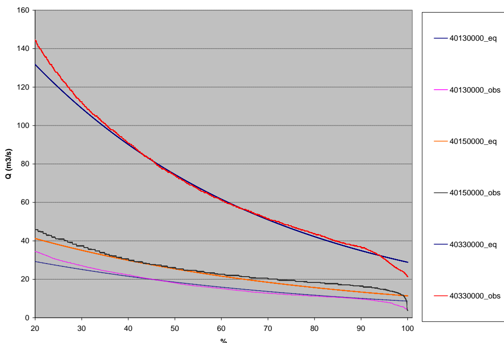
Figura 54 – Ajuste da equação exponencial às curvas de permanência da região homogênea I.
