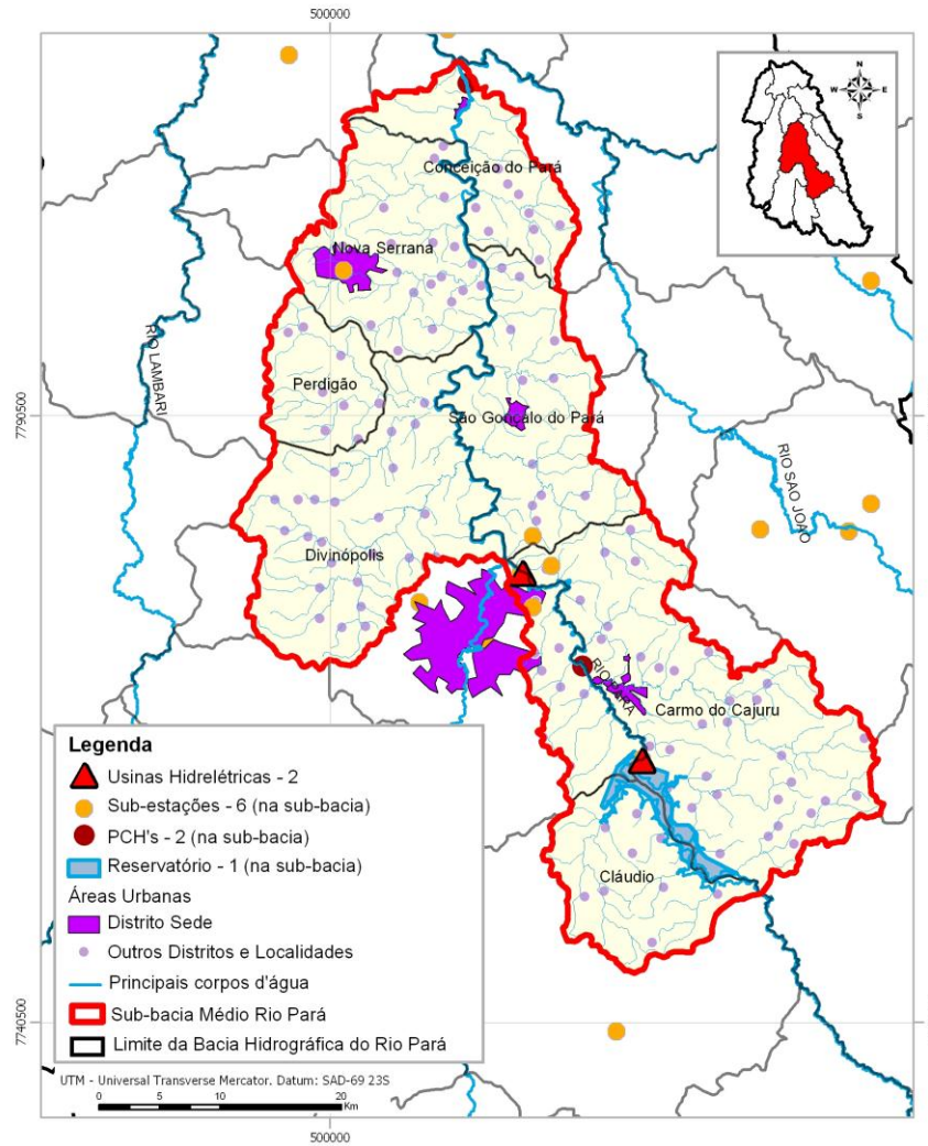
Figura 89 – Geração de energia Sub-bacia Médio Rio Pará
