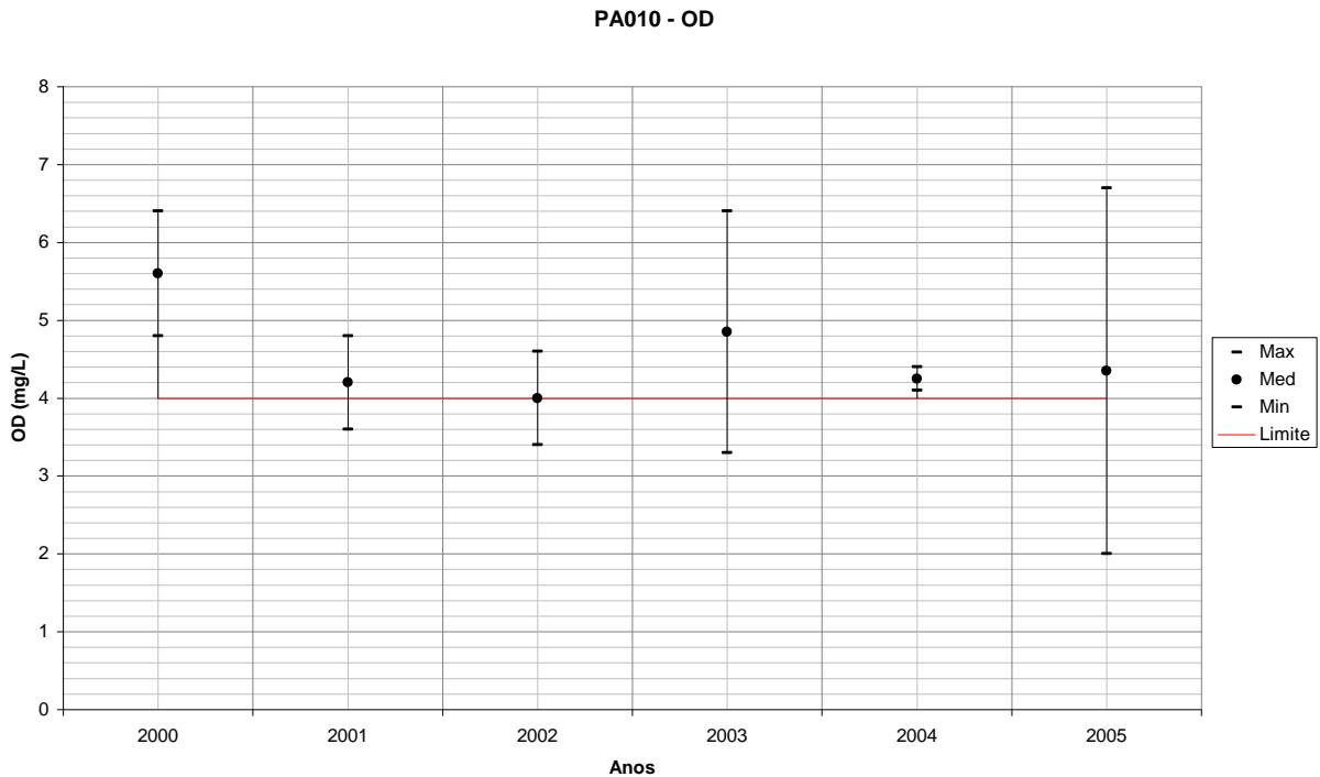
Figura 192 – Variação de OD para PA010 em relação ao período seco de cada ano monitorado. Fonte: IGAM. Processamento TESE Tecnologia em Sistemas Espaciais Ltda.
