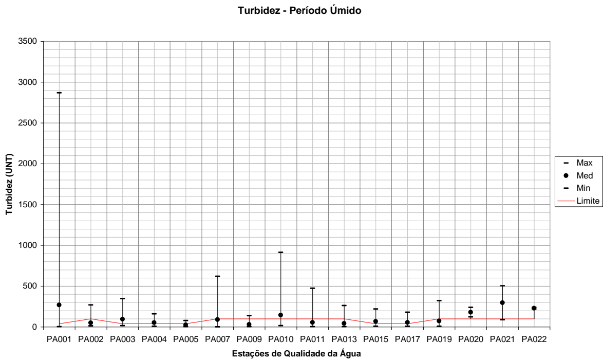
Figura 156 – Variação da Turbidez para todas as estações de qualidade da água em relação a todo o período úmido.
