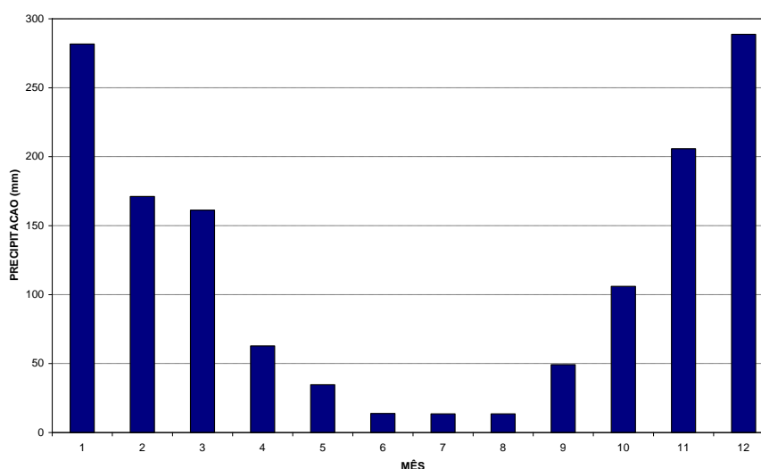
Figura 43 – Precipitação Média Mensal na Bacia Hidrográfica do Rio Pará
