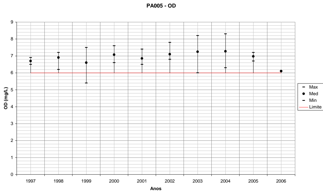
Figura 168 – Variação de OD para PA005 em todos os anos monitorados.
