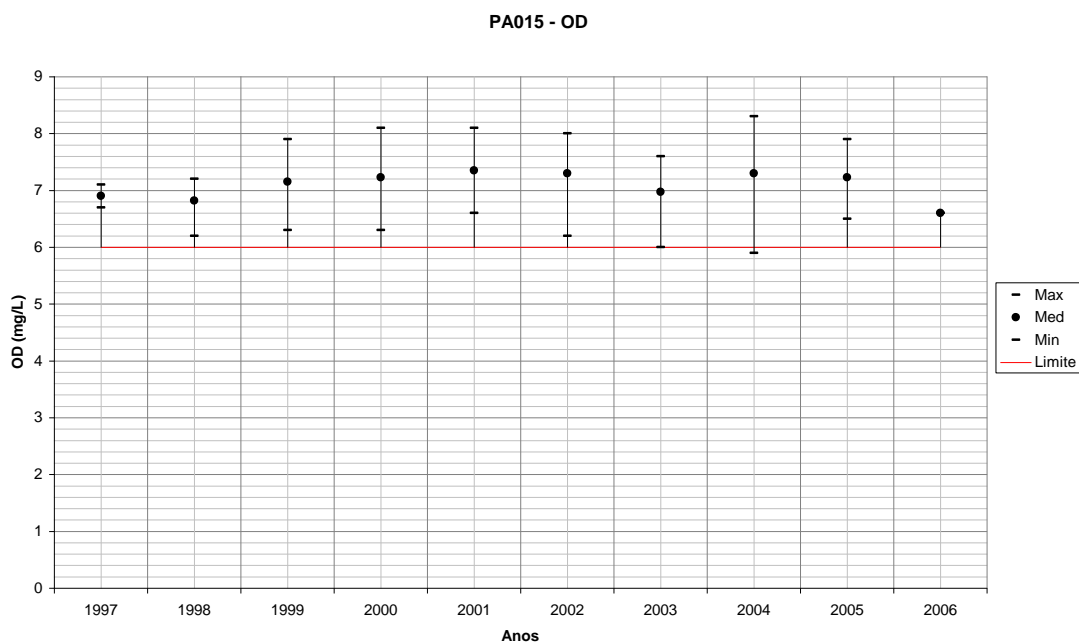
Figura 237 – Variação de OD para PA015 em todos os anos monitorados.
