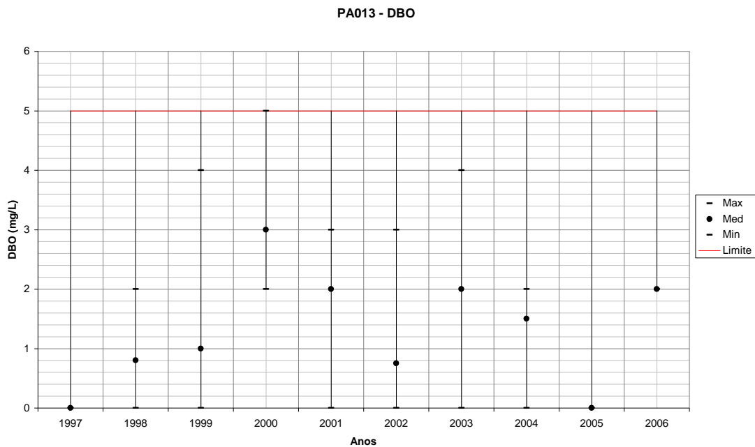
Figura 277 – Variação de DBO para PA013 em todos os anos monitorados.
