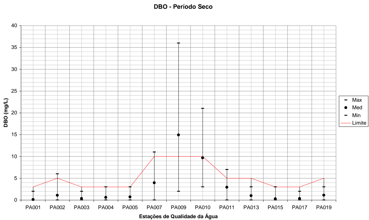
Figura 100 – Variação de DBO para todas as estações de qualidade da água em relação a todo o período seco.
