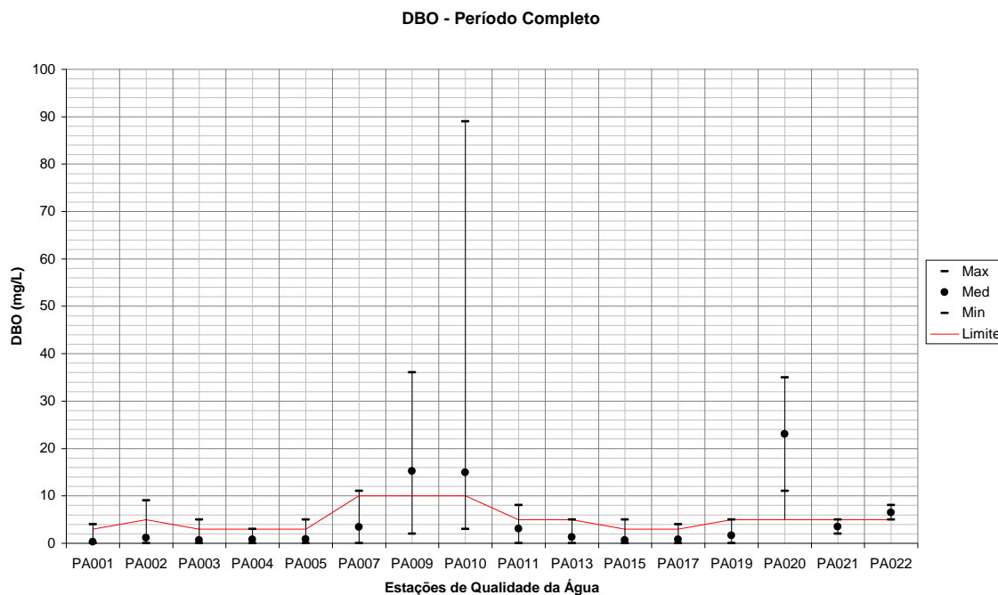
Figura 183 – Variação de DBO para todas as estações de qualidade da água em relação a todo o período monitorado.
