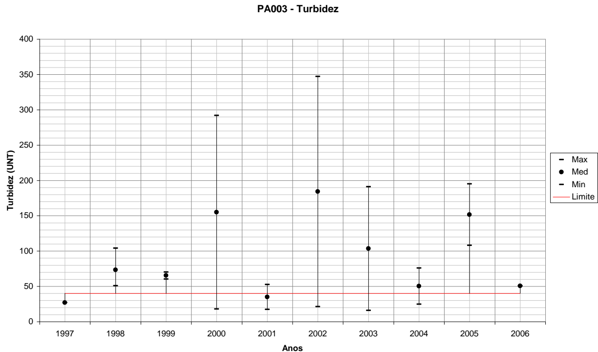
Figura 131 – Variação de Turbidez para PA003 em relação ao período úmido de cada ano monitorado.
