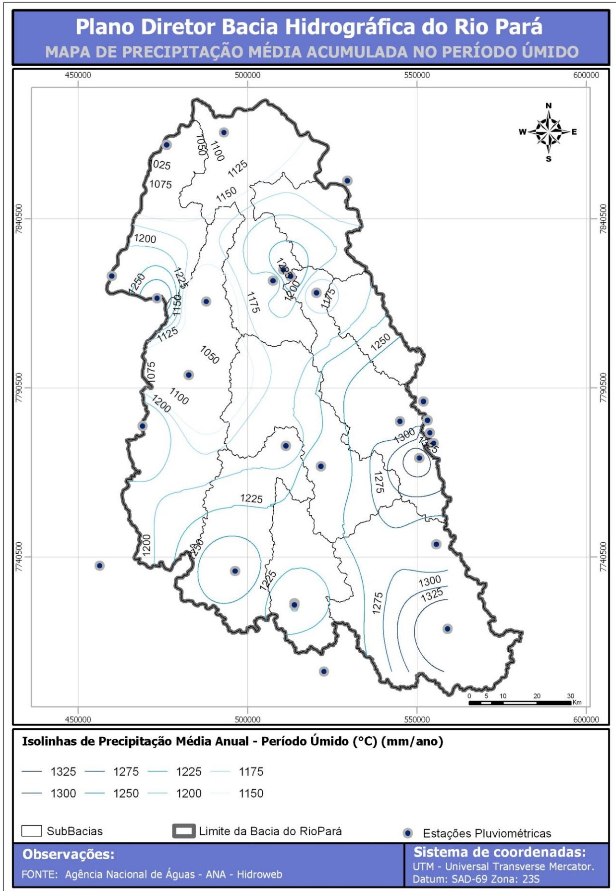
Figura 44 – Isoietas da precipitação média acumulada no período úmido.
