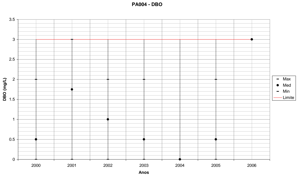
Figura 133 – Variação de DBO para PA004 em todos os anos monitorados.
