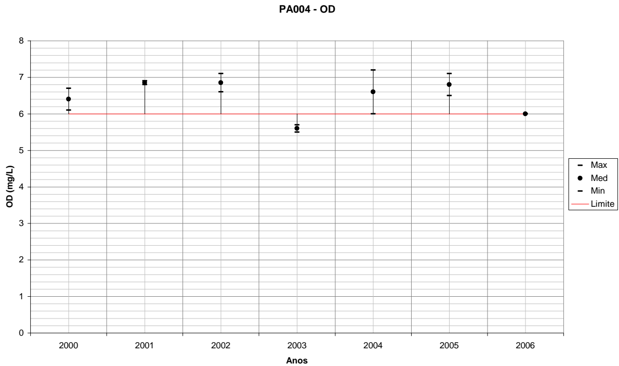
Figura 148 – Variação de OD para PA004 em relação ao período úmido de cada ano monitorado.
