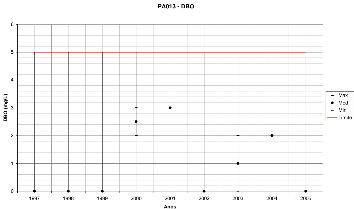
Figura 280 – Variação de DBO para PA013 em relação ao período seco de cada ano monitorado.
