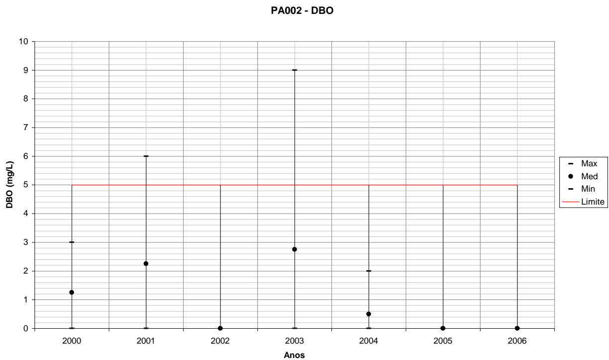
Figura 98 – Variação de DBO para PA002 em todos os anos monitorados.
