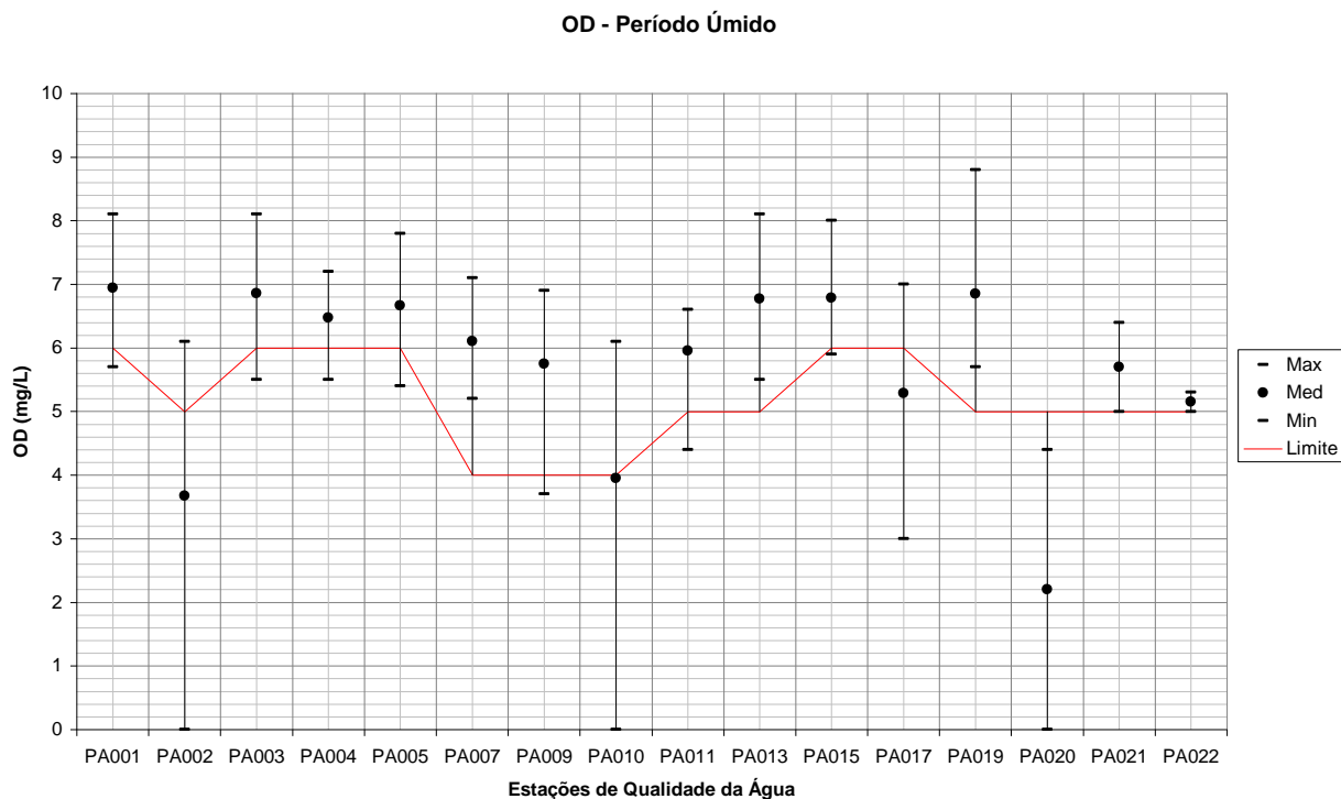
Figura 147 – Variação de OD para todas as estações de qualidade da água em relação a todo o período úmido.
