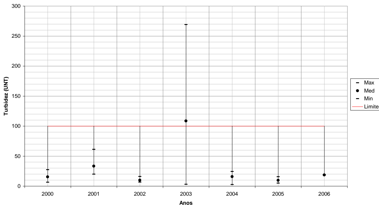
Figura 122 – Variação de Turbidez para PA002 em todos os anos monitorados.
