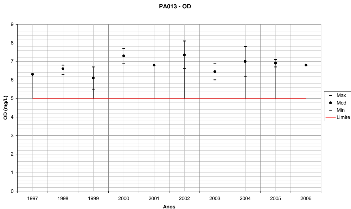
Figura 292 – Variação de OD para PA013 em relação ao período úmido de cada ano monitorado.
