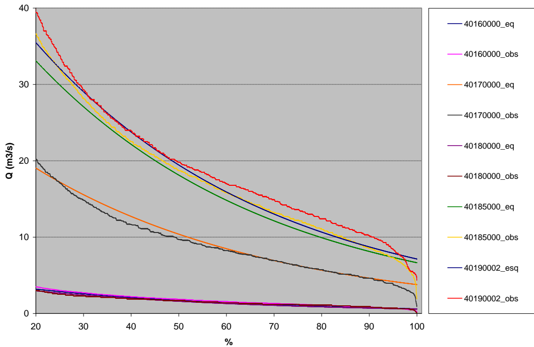
Figura 55 – Ajuste da equação exponencial às curvas de permanência da região homogênea II.
