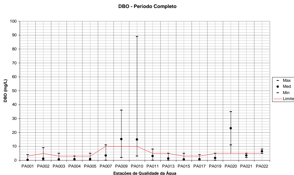
Figura 201 – Variação de DBO para todas as estações de qualidade da água em relação a todo o período monitorado.
