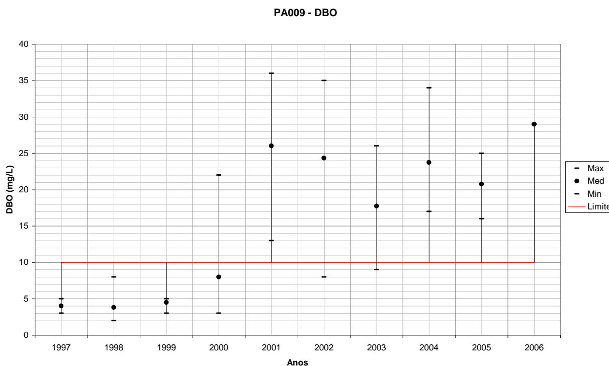
Figura 202 – Variação de DBO para PA009 em todos os anos monitorados.
