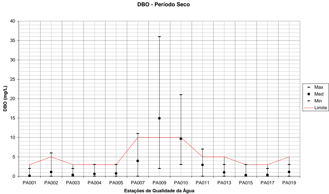
Figura 135 – Variação de DBO para todas as estações de qualidade da água em relação a todo o período seco.
