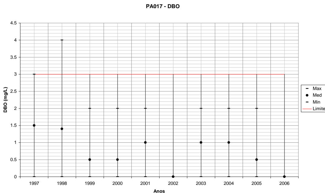
Figura 253 – Variação de DBO para PA017 em todos os anos monitorados.
