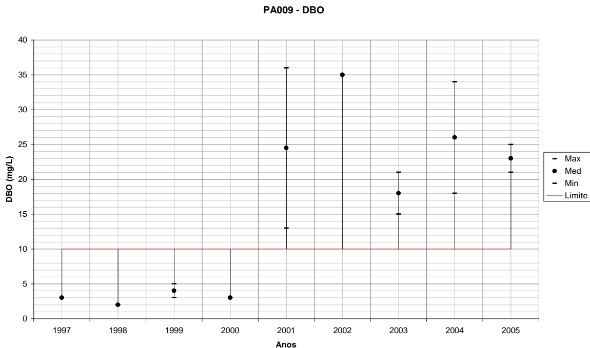
Figura 205 – Variação de DBO para PA009 em relação ao período seco de cada ano monitorado. Fonte: IGAM. Processamento TESE Tecnologia em Sistemas Espaciais Ltda.
