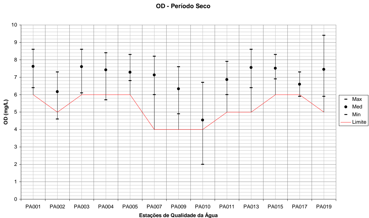
Figura 239 – Variação de OD para todas as estações de qualidade da água em relação a todo o período seco.
