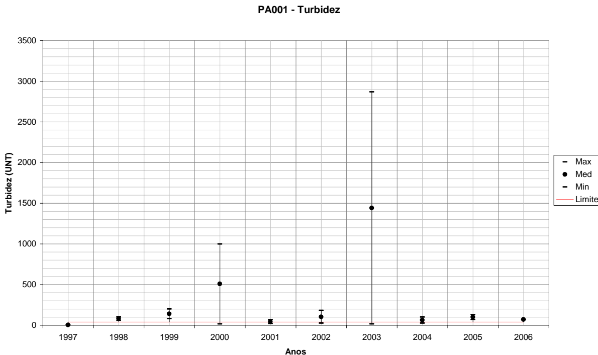
Figura 129 – Variação de Turbidez para PA001 em relação ao período úmido de cada ano monitorado.
