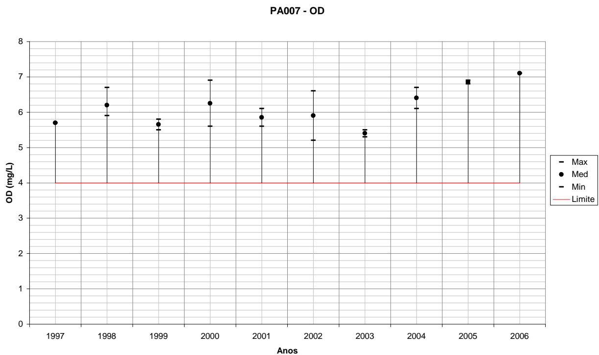
Figura 149 – Variação de OD para PA007 em relação ao período úmido de cada ano monitorado.
