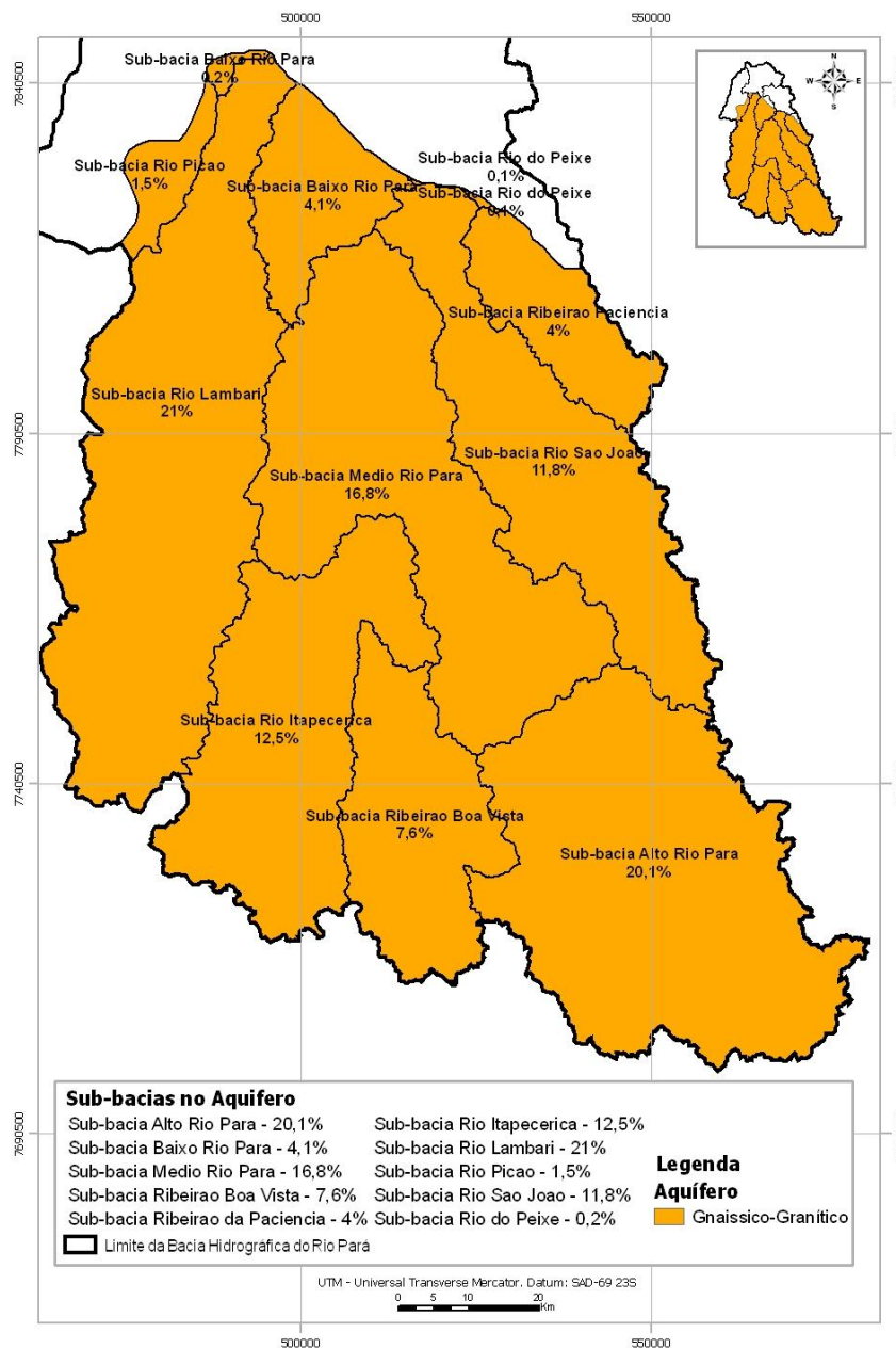
Figura 64 – Abrangência do Sistema Aquífero Gnáissico-Granítico na Bacia hidrográfica do Rio Pará
