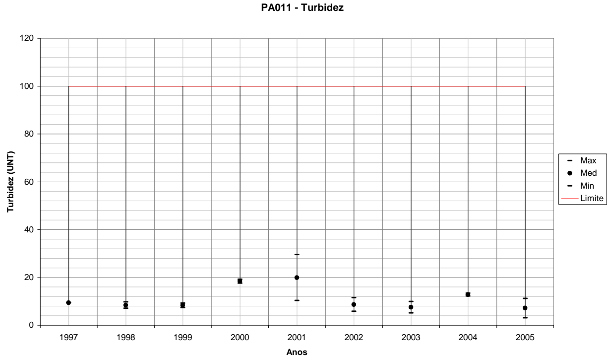
Figura 224 – Variação de Turbidez para PA011 em relação ao período seco de cada ano monitorado.
