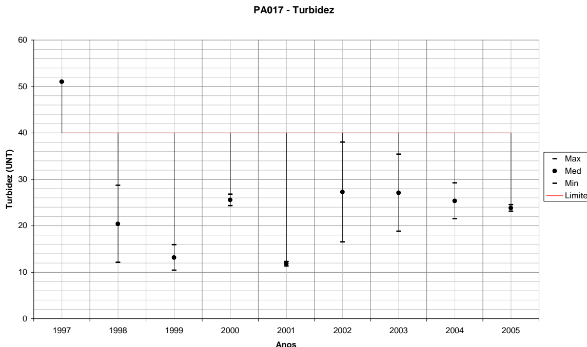
Figura 272 – Variação de Turbidez para PA017 em relação ao período seco de cada ano monitorado.
