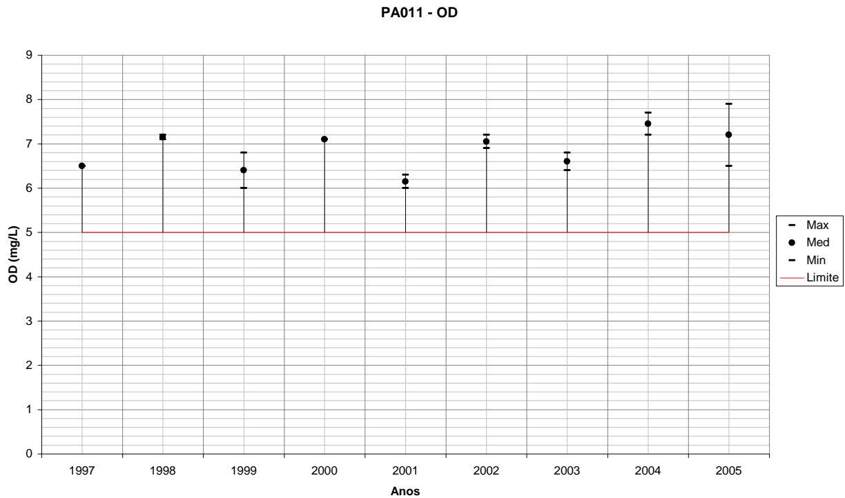
Figura 215 – Variação de OD para PA011 em relação ao período seco de cada ano monitorado.
