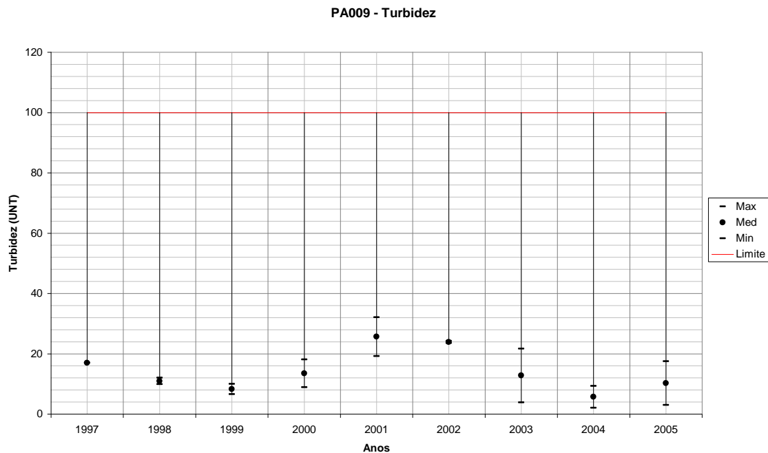
Figura 223 – Variação de Turbidez para PA009 em relação ao período seco de cada ano monitorado.
