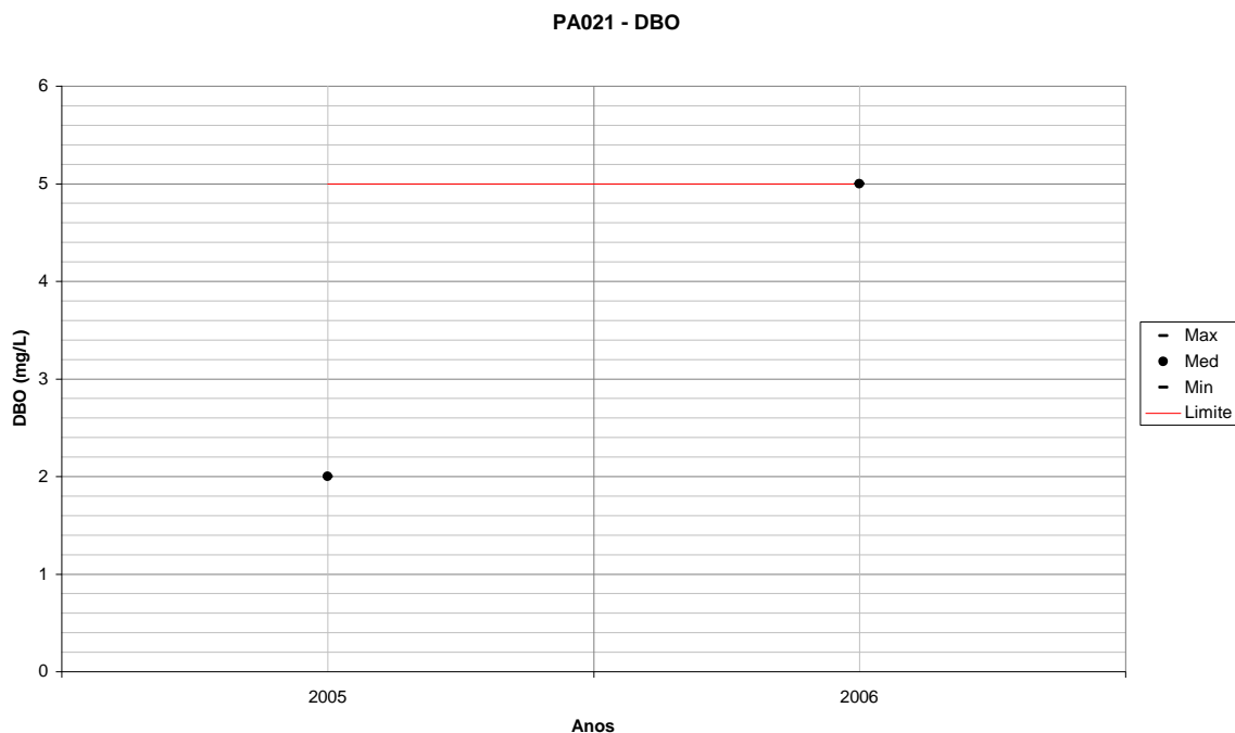
Figura 259 – Variação de DBO para PA021 em relação ao período úmido de cada ano monitorado. Fonte: IGAM. Processamento TESE Tecnologia em Sistemas Espaciais Ltda.
