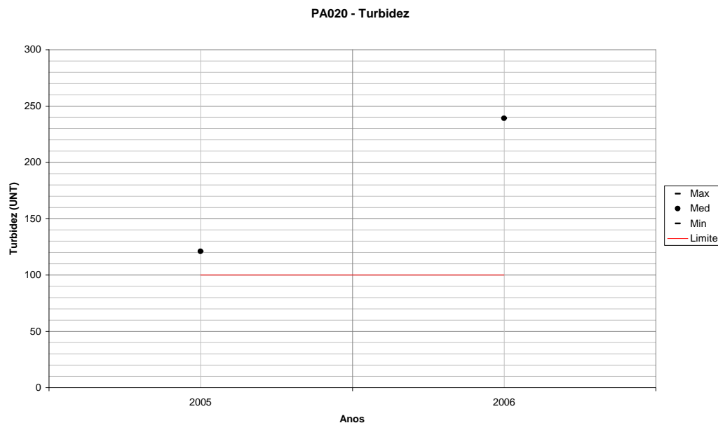
Figura 182 – Variação de Turbidez para PA020 em relação ao período úmido de cada ano monitorado.
