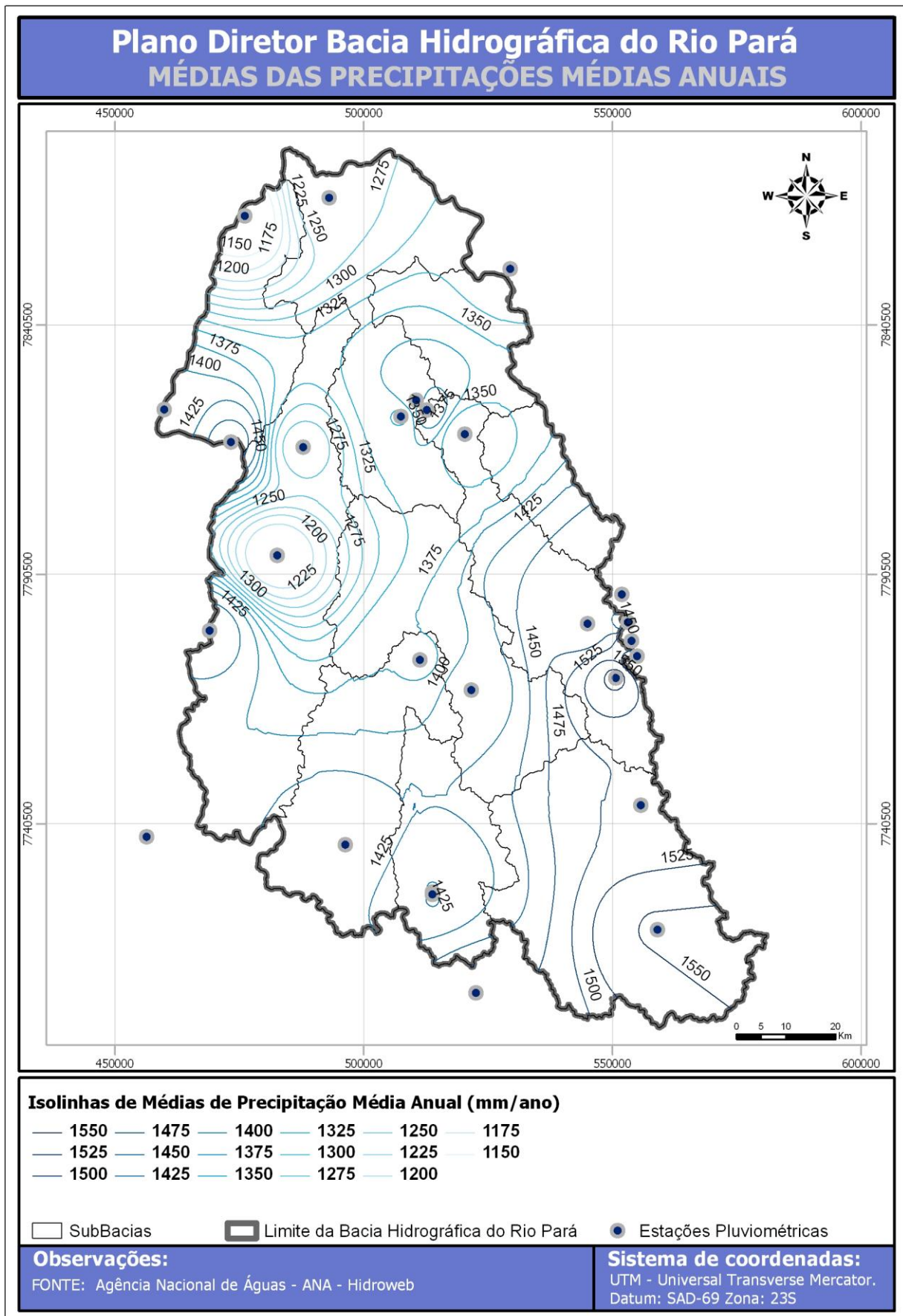
Figura 39 – Isoietas da precipitação média anual
