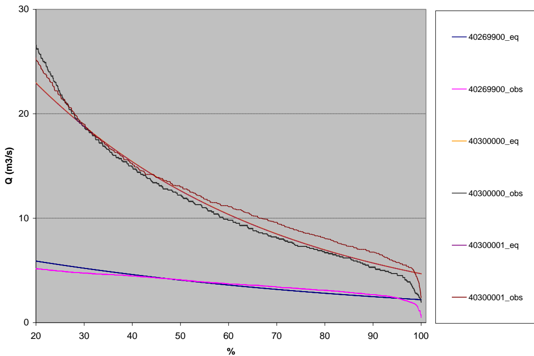
Figura 56 – Ajuste da equação exponencial às curvas de permanência da região homogênea III.
