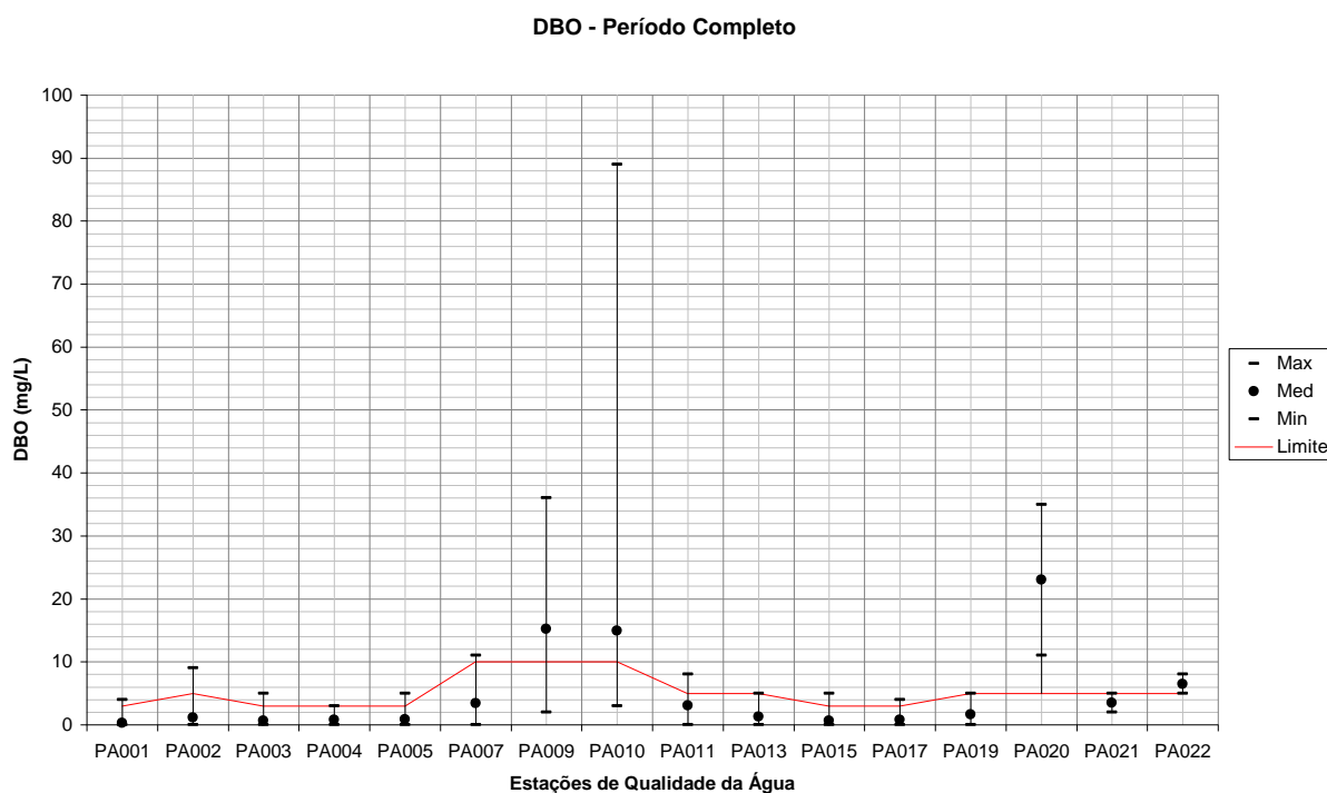
Figura 159 – Variação de DBO para todas as estações de qualidade da água em relação a todo o período monitorado.
