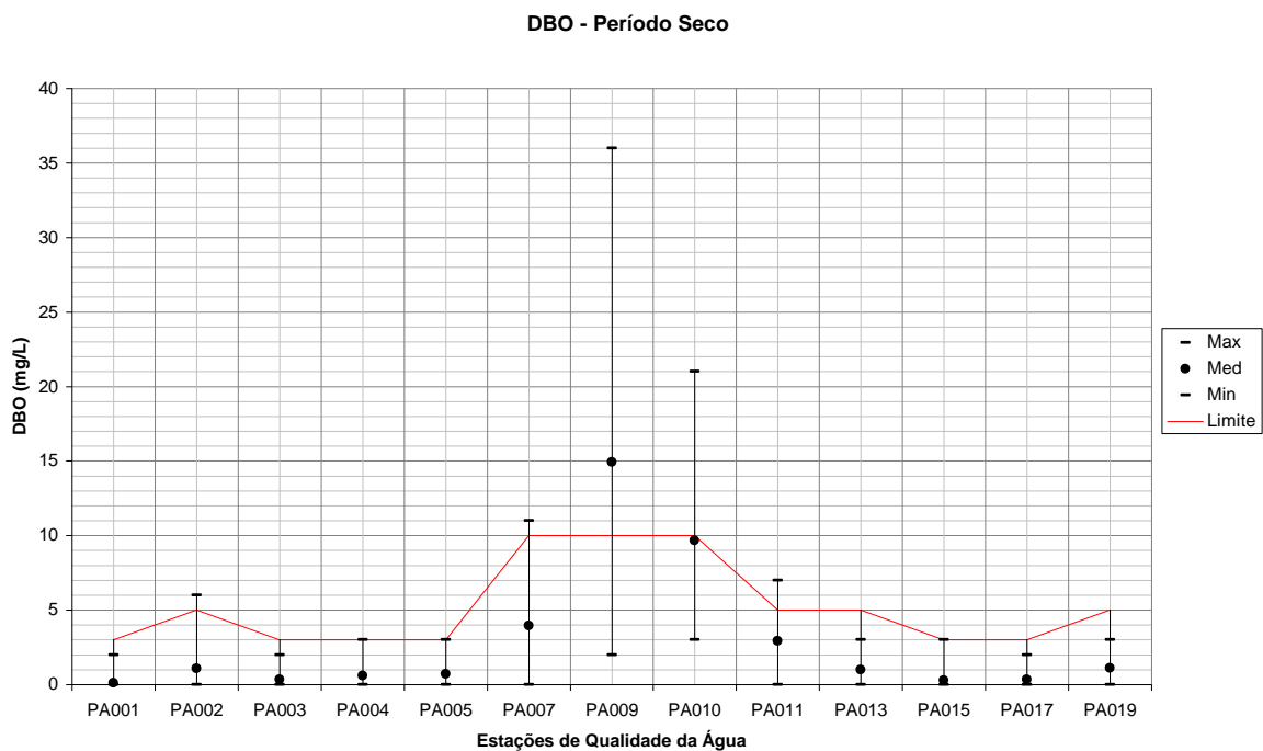
Figura 204 – Variação de DBO para todas as estações de qualidade da água em relação a todo o período seco.
