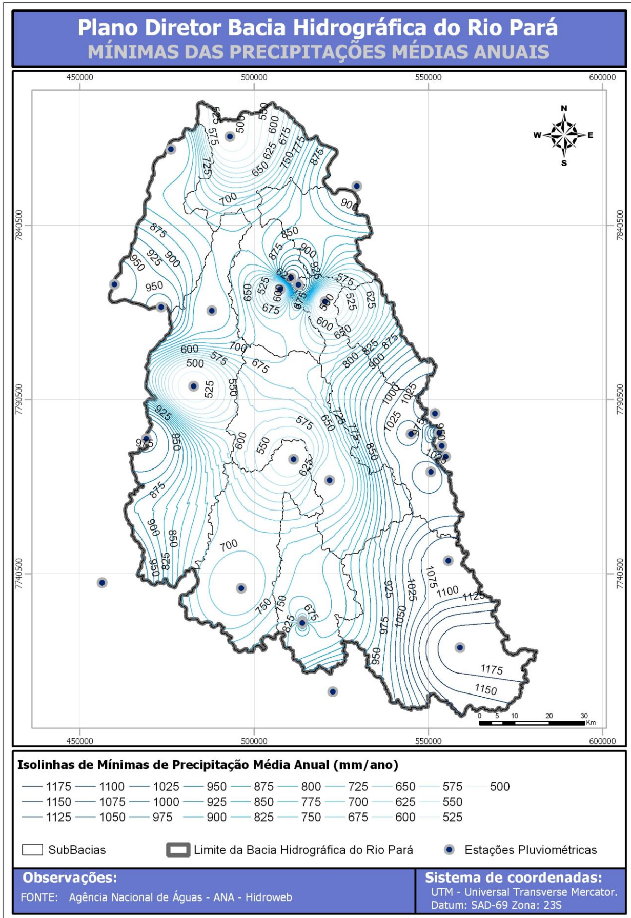
Figura 41 – Isoietas da precipitação média anual mínima
