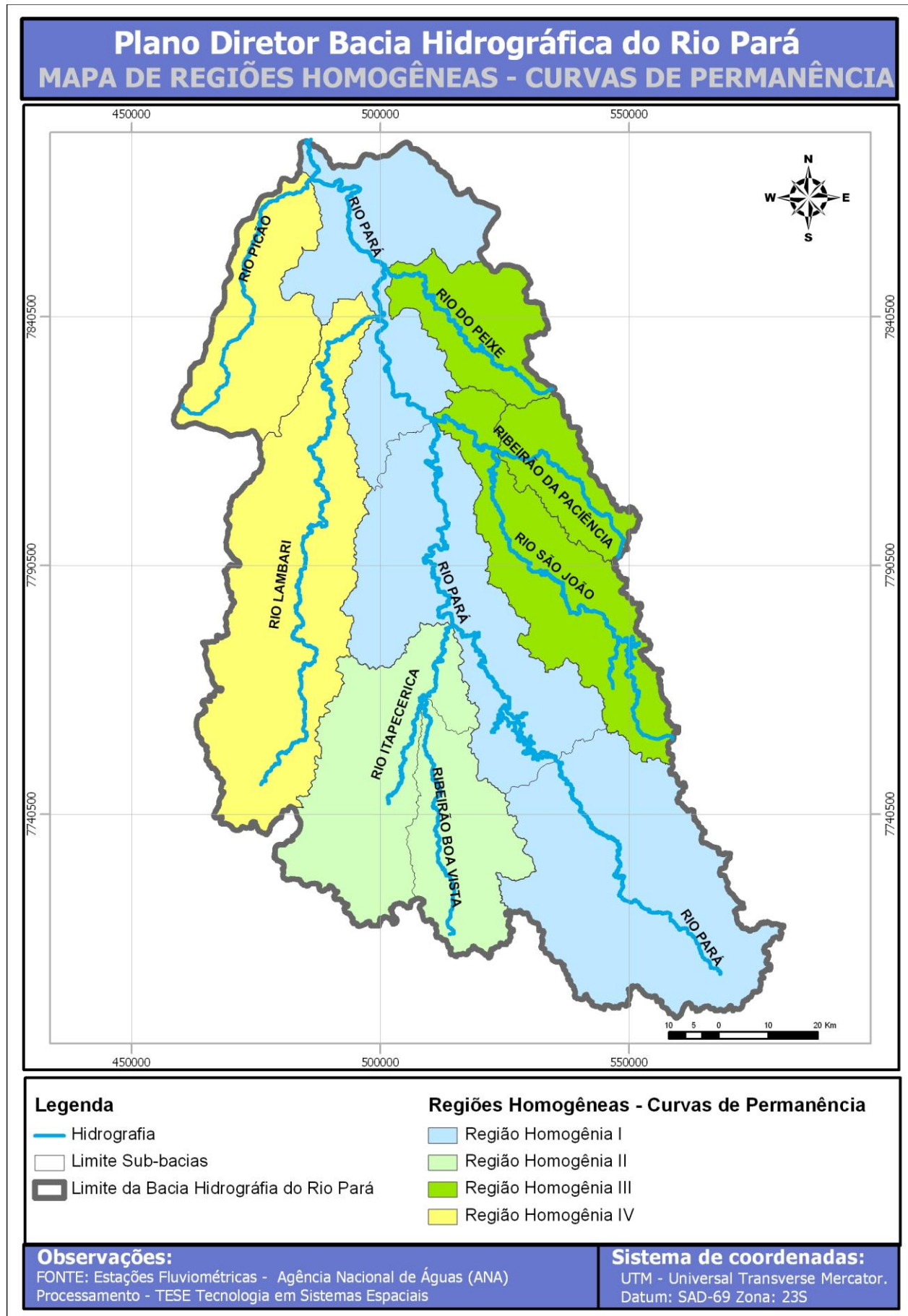
Figura 53 – Regiões homogêneas para as curvas de permanência
