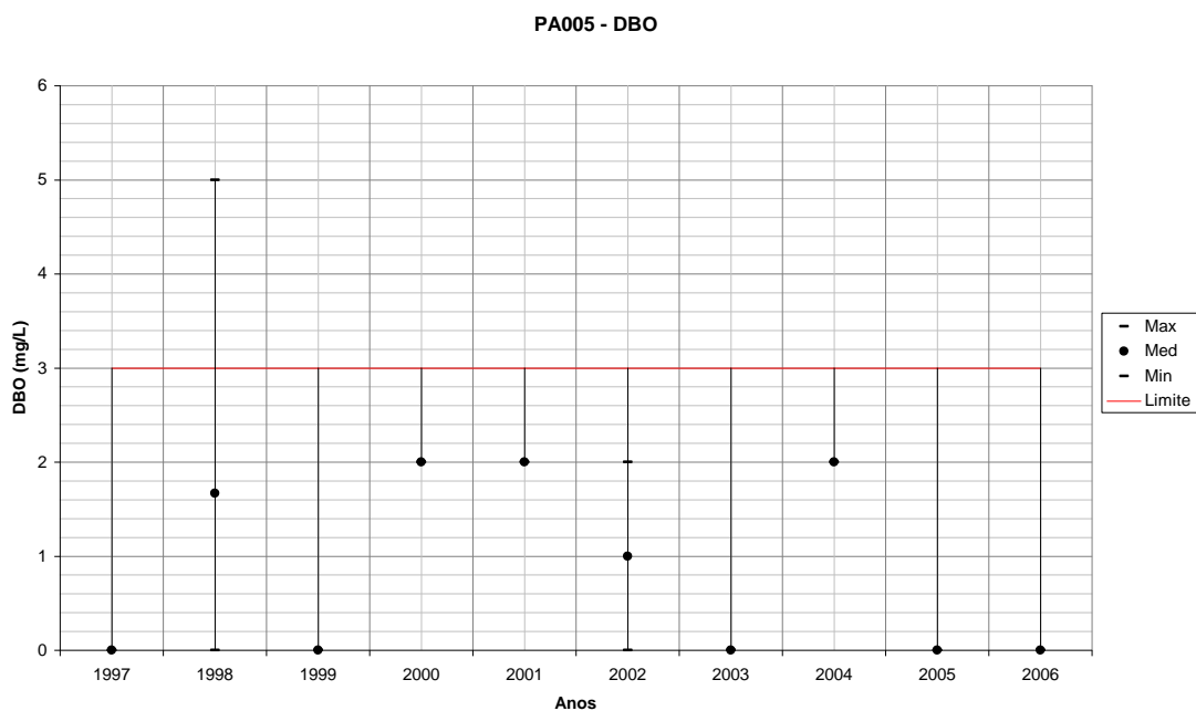
Figura 165 – Variação de DBO para PA005 em relação ao período úmido de cada ano monitorado.
