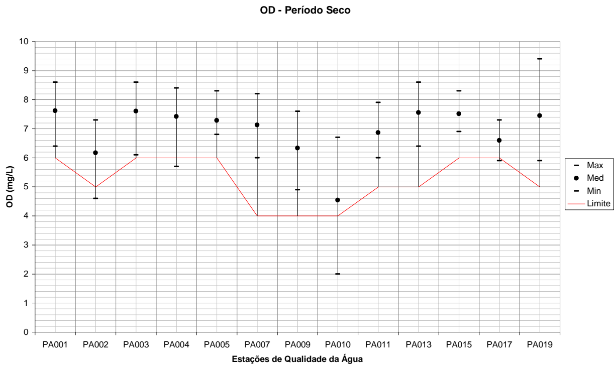
Figura 213 – Variação de OD para todas as estações de qualidade da água em relação a todo o período seco.
