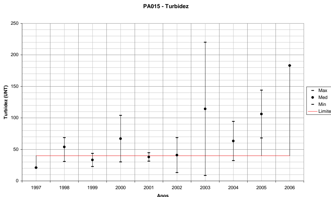
Figura 250 – Variação de Turbidez para PA015 em relação ao período úmido de cada ano monitorado.
