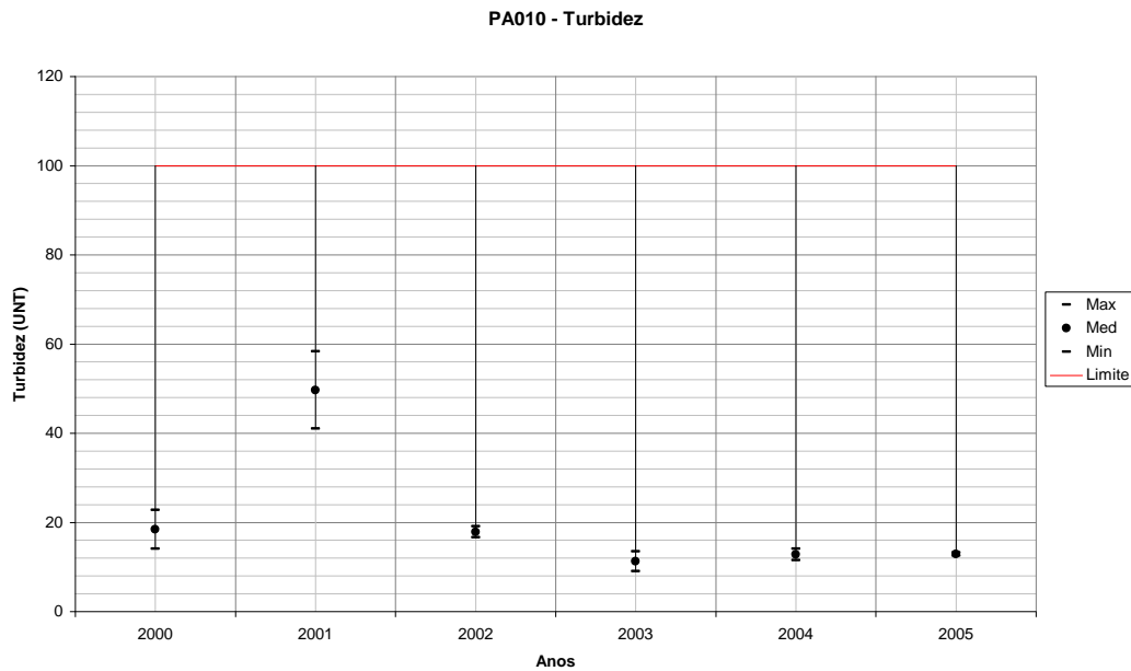
Figura 198 – Variação de Turbidez para PA010 em relação ao período seco de cada ano monitorado.
