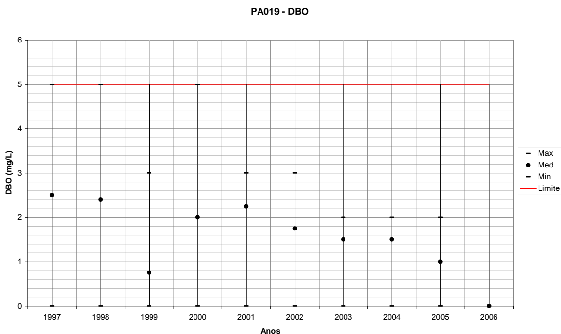
Figura 278 – Variação de DBO para PA019 em todos os anos monitorados.
