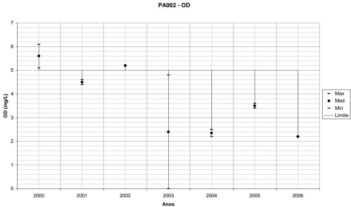
Figura 118 – Variação de OD para PA002 em relação ao período úmido de cada ano monitorado.
