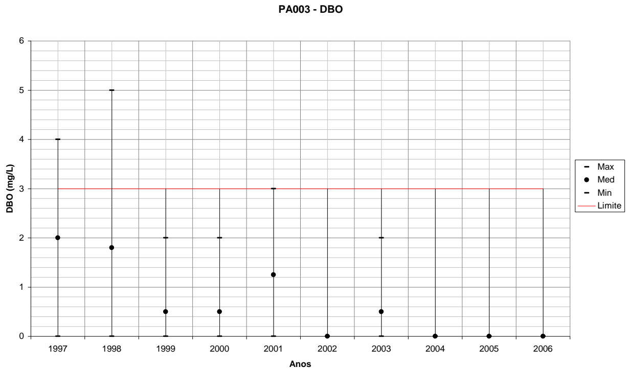
Figura 99 – Variação de DBO para PA003 em todos os anos monitorados.
