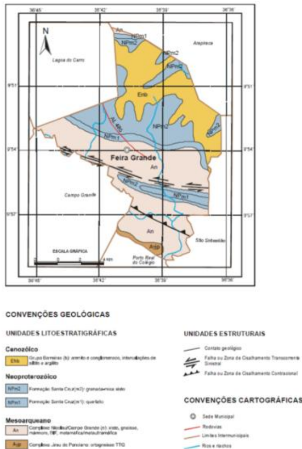
Figura 2 – Mapa Geológico do município de Feira Grande
