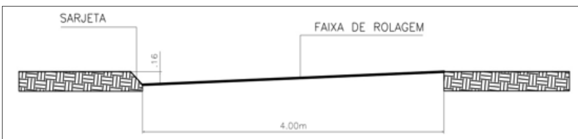
Figura 22 - Esquema da estrada considerando uma largura média de 4 metros de largura, 4% de declividade e sarjeta com 16 cm de profundidade.
